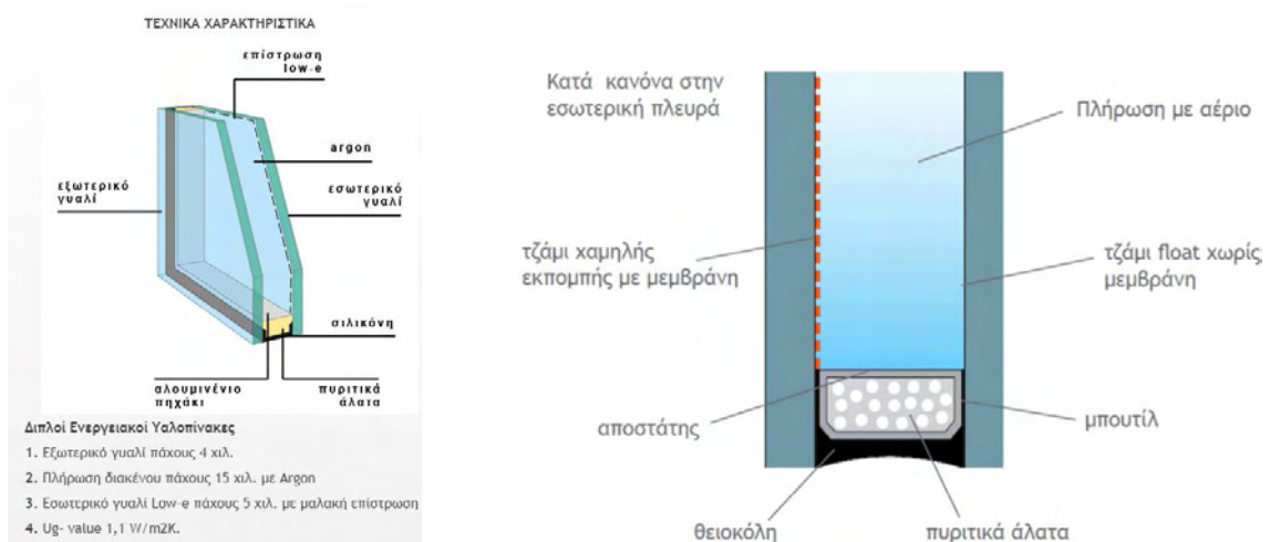
Εικόνα 2.4: Τομή υαλοπίνακα,
