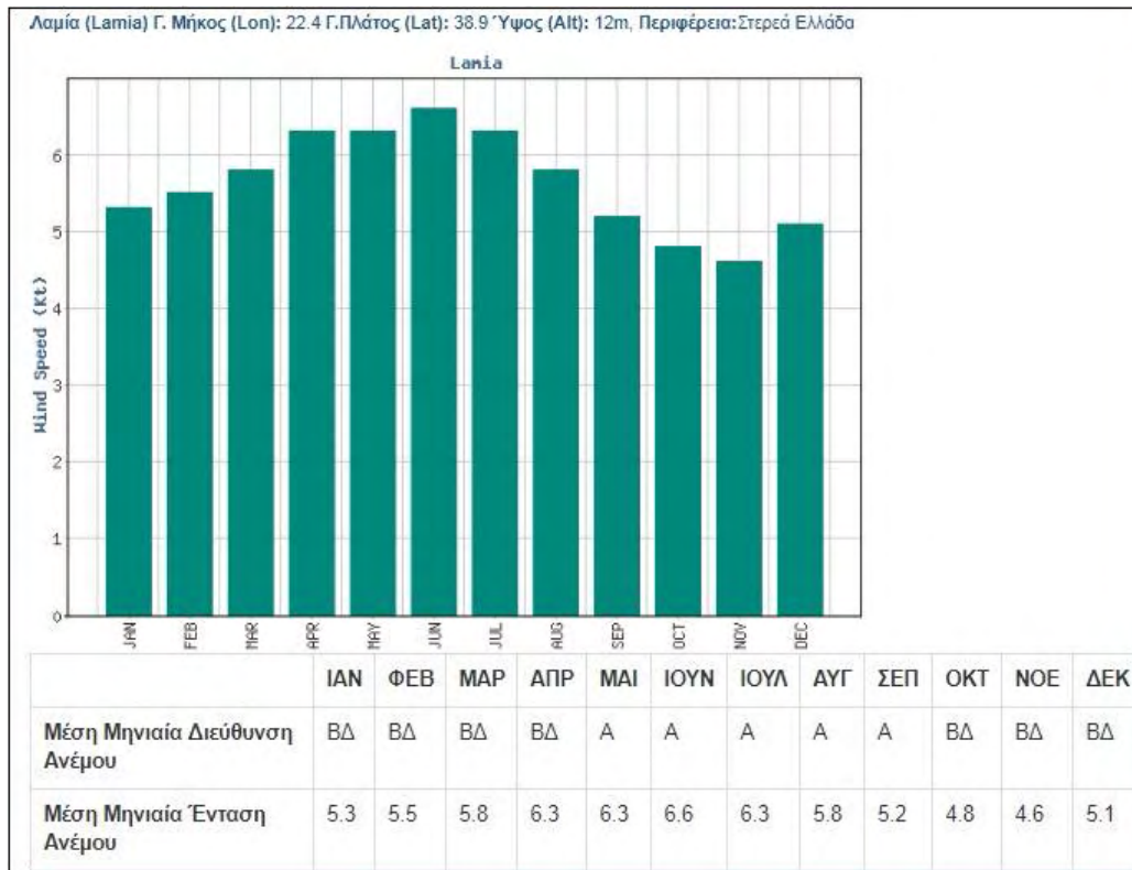
Εικόνα 4.9., Διάγραμμα ετήσιας διακύμανσης ανέμου, (Πηγή: http://www.hnms.gr/emv/el/climatology/climatology_city?perifereia=Sterea&poli=Lamia )
