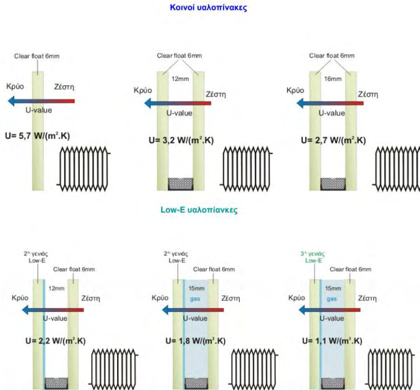
Εικόνα 2.6: Εξέλιξη του συντελεστή θερμοπερατότητας υαλοστασίων (κοινών και low-e) (Πηγή: http://www.prismaglass.gr/dat/prisma_storage/dat/67AEE251/news19.pdf )
