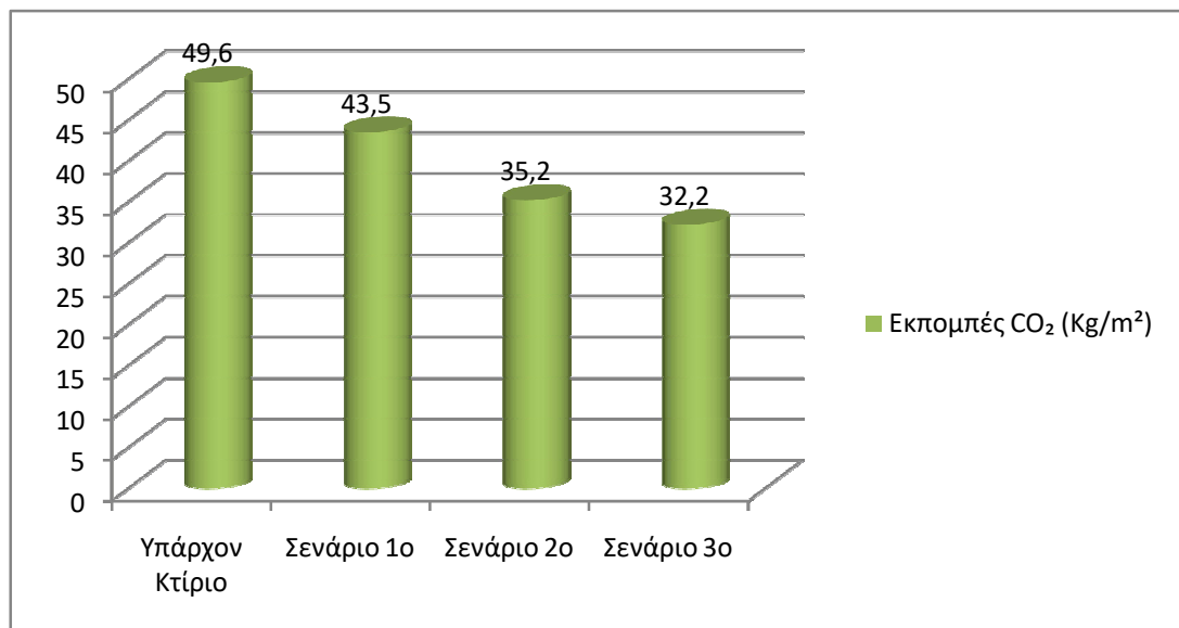
Εικόνα 5.7 Εκπομπές CO 2 ( kg/m^2 )
