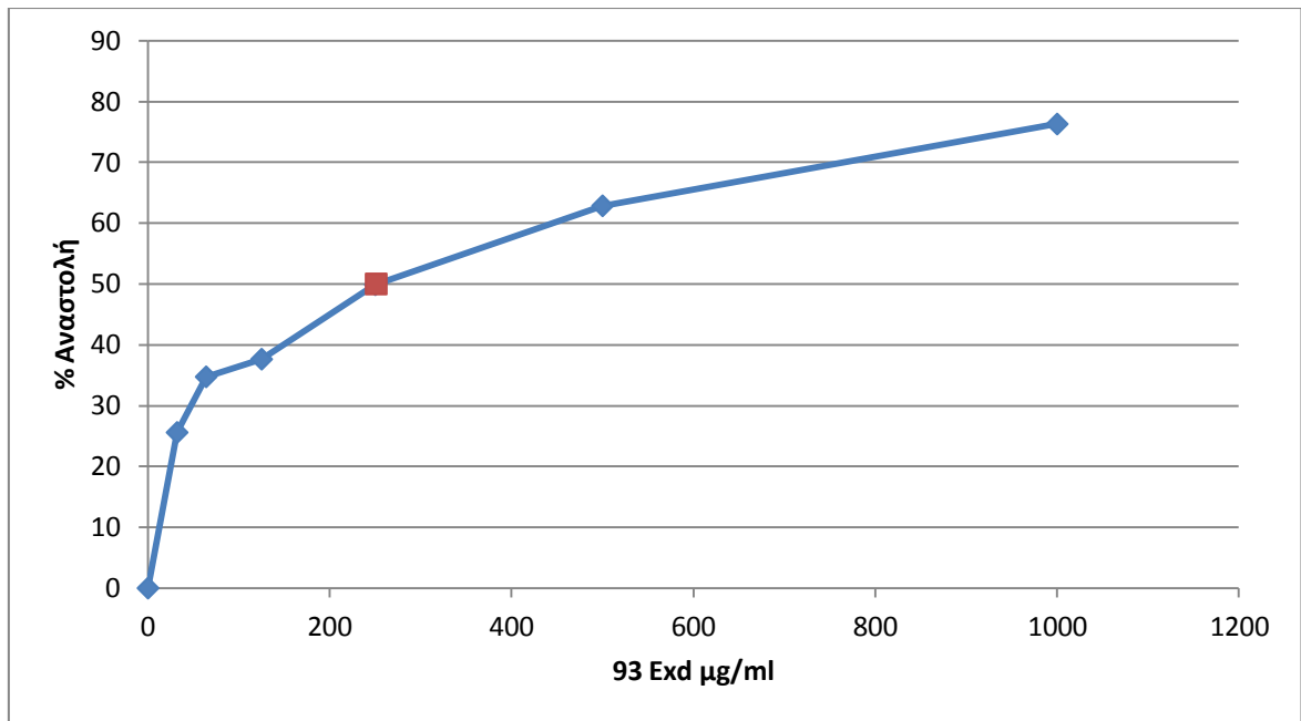
Διάγραμμα 4.4.2. Το διάγραμμα απεικονίζει την % αναστολή (εξουδετέρωση) της ρίζας OH - από το εκχύλισμα 93 Ecd ( Conium divaricatum ).
