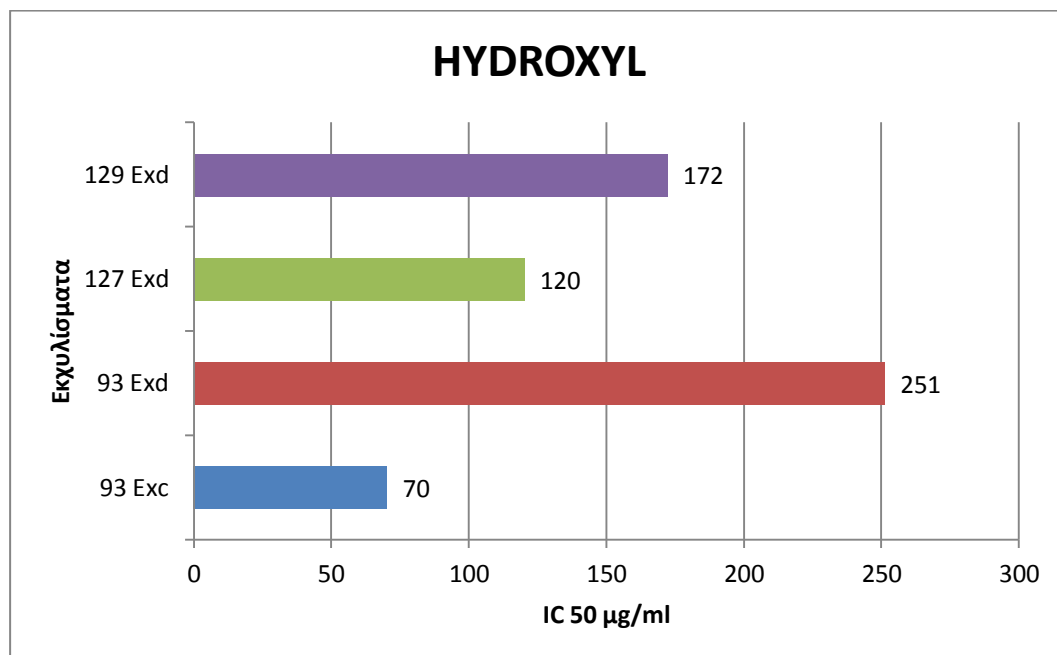
Διάγραμμα 4.4.5. Απεικονίζονται οι τιμές IC 50 που προκύπτουν για την εξουδετέρωση της ρίζας OH από τα υπό εξέταση εκχυλίσματα
