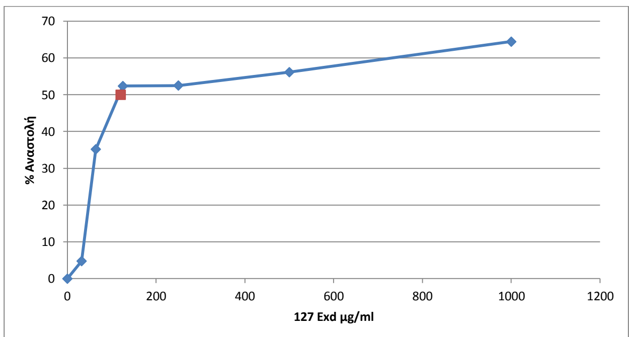
Διάγραμμα 4.4.3. Το διάγραμμα απεικονίζει την % αναστολή (εξουδετέρωση) της ρίζας OH - από το εκχύλισμα 127 Ecd ( Artemisia arborescens ).
