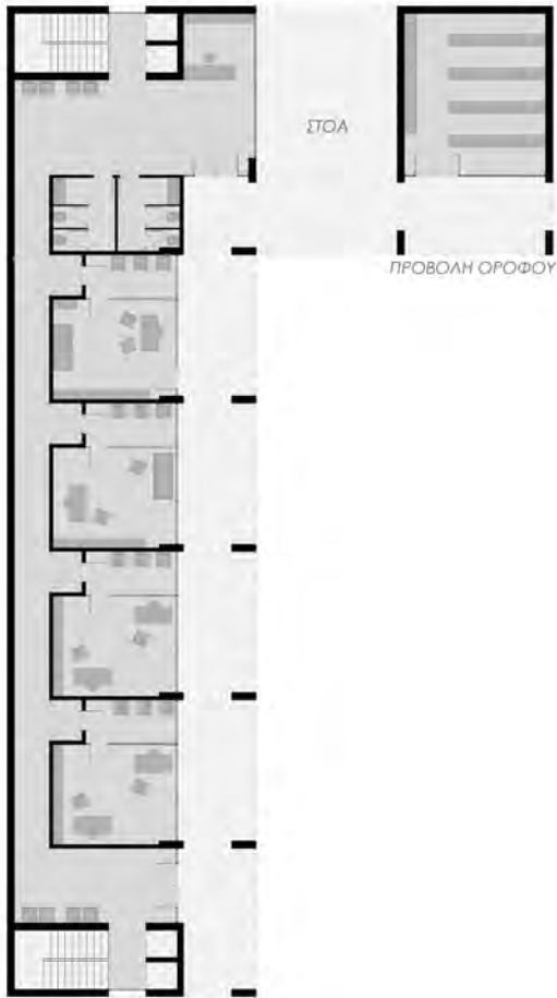
κάνοψη ισογείου
