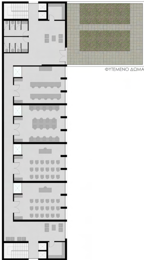
κάτοψη 2ου ορόφου
