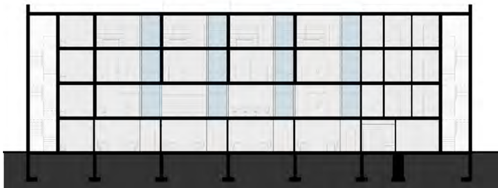
τομή 5-5
