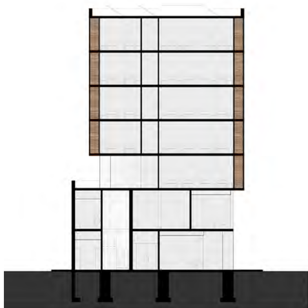
τομή 2-2
