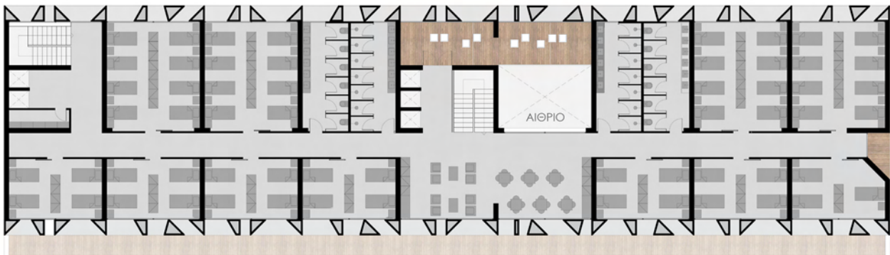
κάτοψη 3,4,5,6ου ορόφου
