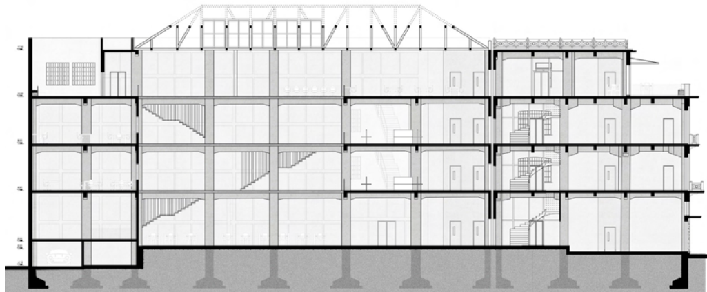
ΤΟΜΗ Α-Α
