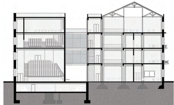
TOMH B-B
