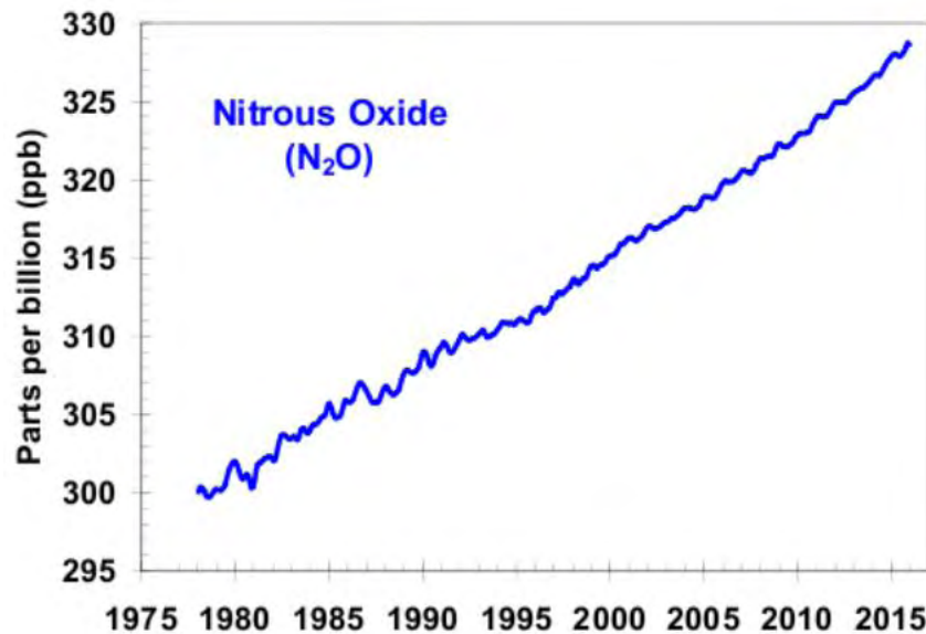
Διάγραμμα 4: Η μεταβολή στη συγκέντρωση του υποξειδίου του αζώτου.
