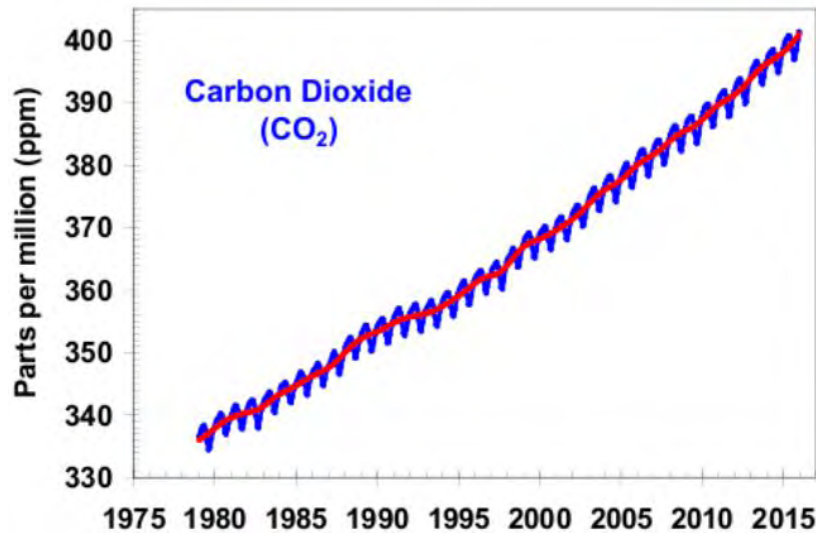
Διάγραμμα 1: Η αύξηση της συγκέντρωσης του διοξειδίου του άνθρακα από το 1975 μέχρι το 2015.
