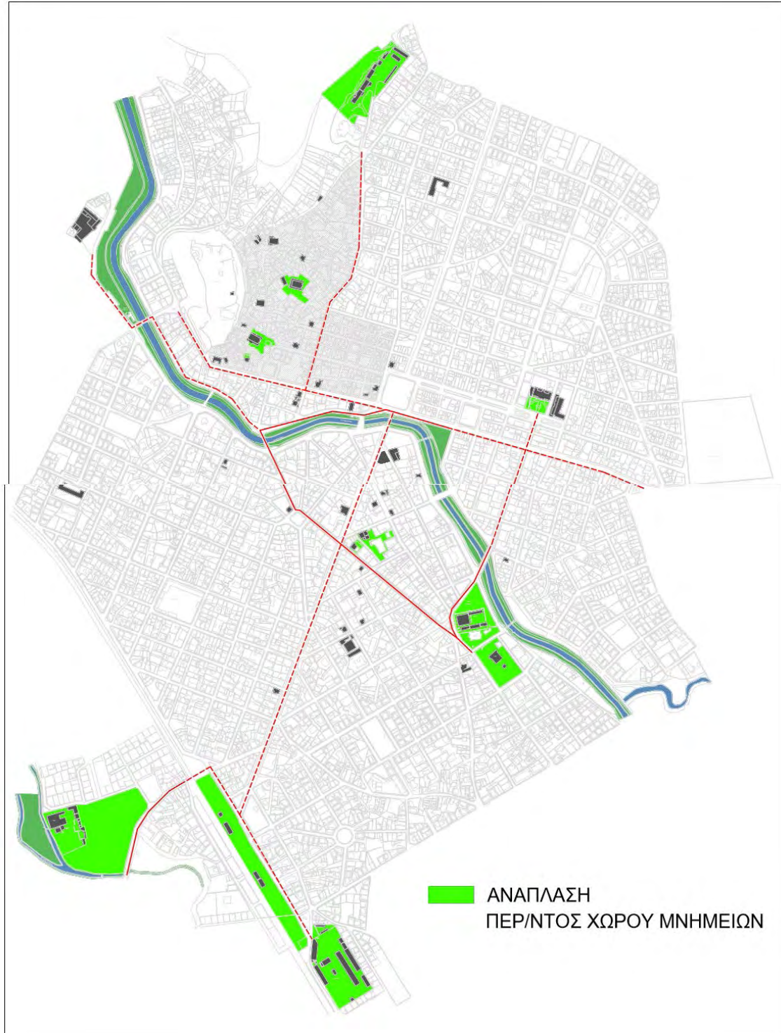
Χάρτης 8. Προτάσεις. (πηγή: ίδια επεξεργασία)
