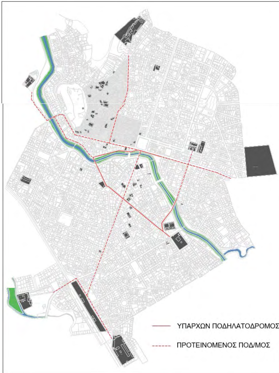
Χάρτης 8. Προτάσεις. (πηγή: ίδια επεξεργασία)
