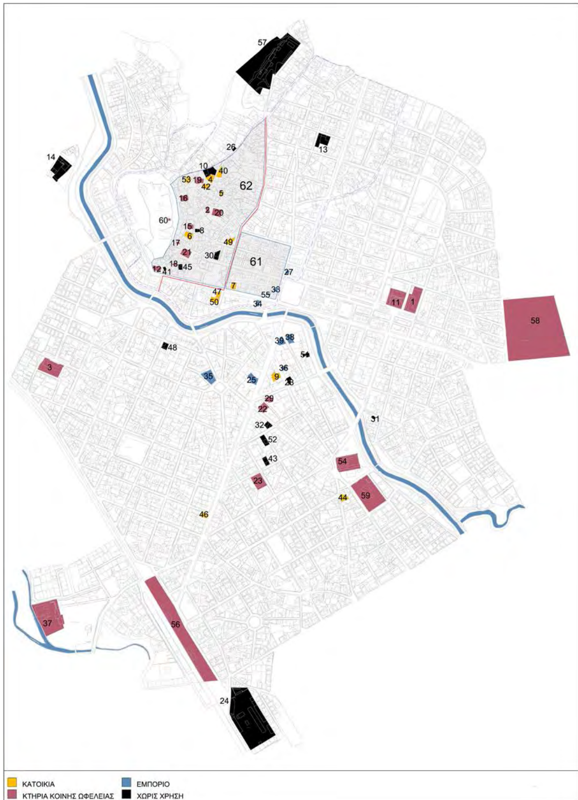
Χάρτης 5. Χωρική απεικόνιση των κτηρίων συναρτήσει της παρούσας χρήσης. (πηγή: ίδια επεξεργασία)
