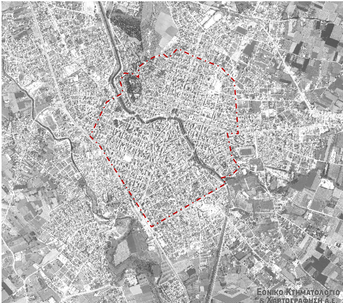
Εικόνα 5. Η περιοχή μελέτης. (πηγή: ίδια επεξεργασία σε χάρτη του Εθνικού Κτηματολογίου)
