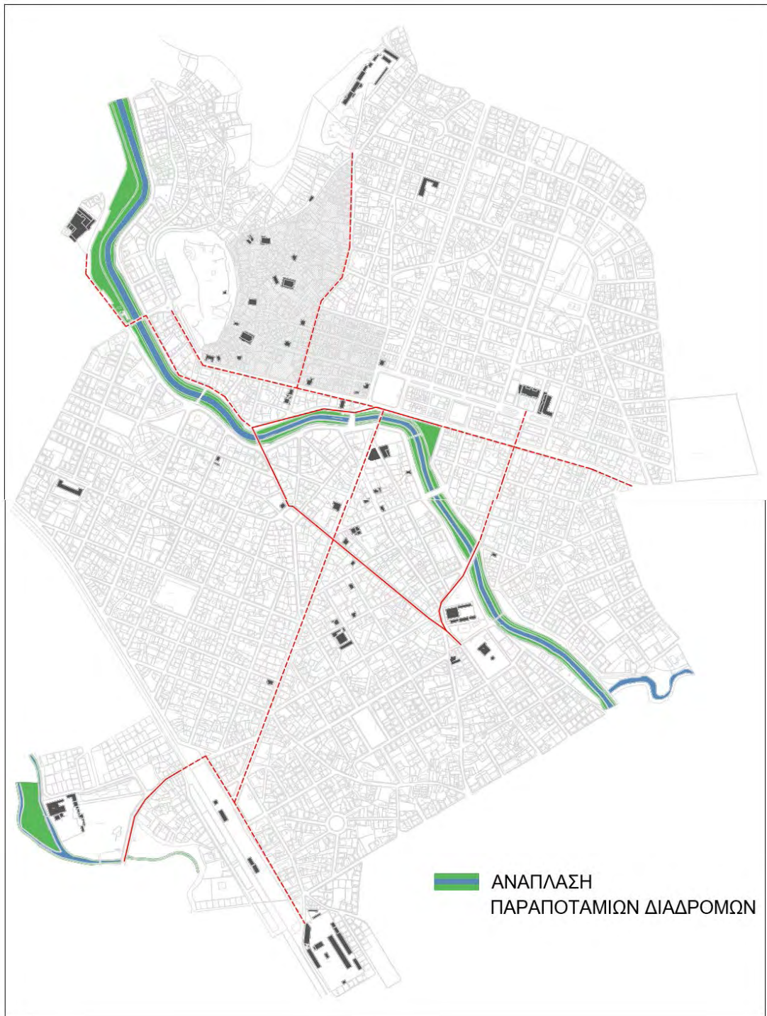
Χάρτης 8. Προτάσεις. (πηγή: ίδια επεξεργασία)
