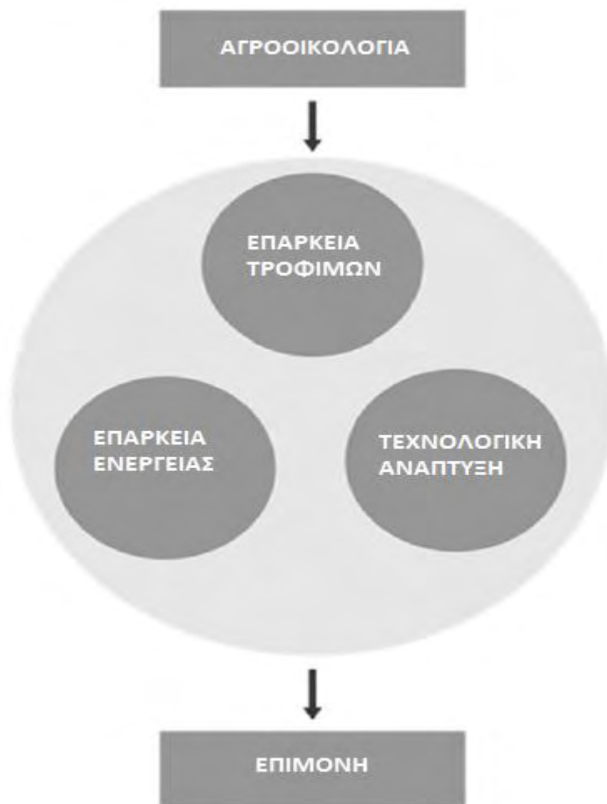
Εικόνα 37: Σχηματική απεικόνιση των τριών θεμέλιων λίθων που απαιτούνται προκειμένου να μπορέσει το κίνημα της αγροικολογίας να καθιερωθεί. Τελευταίο και βασικό στοιχείο είναι η επιμονή όσων αποφασίσουν να συμμετέχουν σε αυτή την προσπάθεια (επιστήμονες, αγρότες ,κοινωνίες) (Altieri et al. 2012).
