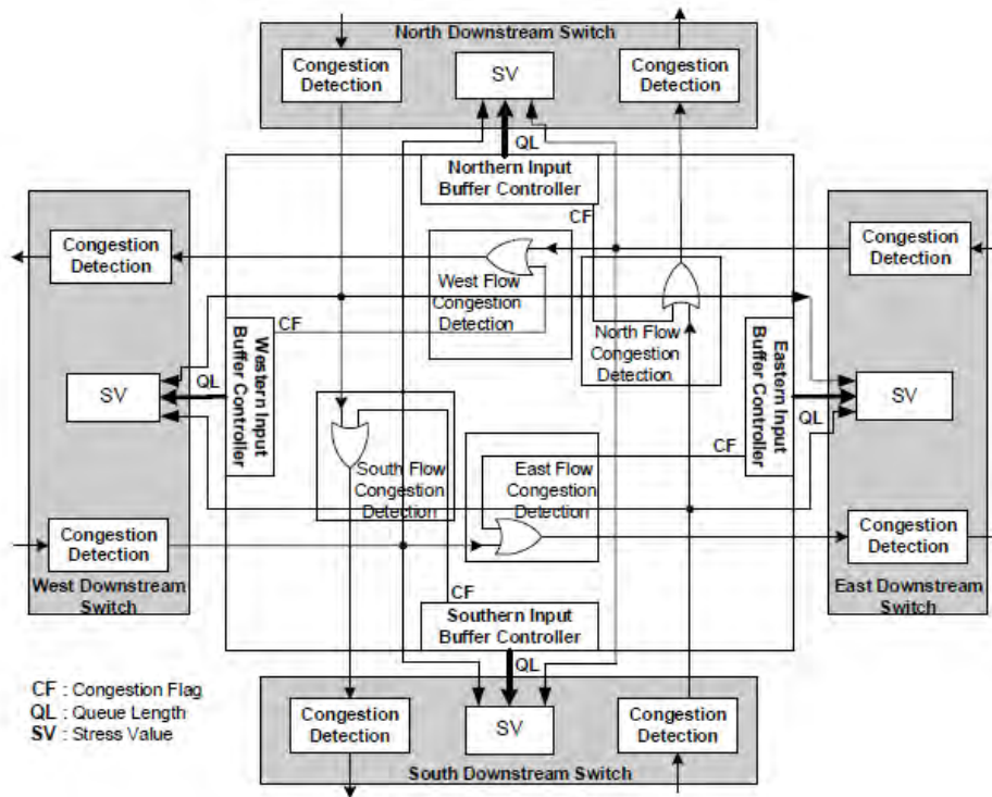
Εικόνα 2.6 Εφαρμογή δρομολογητή EDXY
