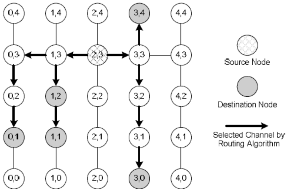
Εικόνα 2.14 Παράδειγμα tree-based multicast αλγορίθμου 5×5 σε 2D-mesh.
