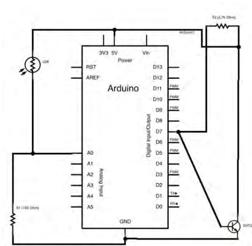
Σχήμα 8-3 : Το σχηματικό του κυκλώματος. Μπορείτε να δείτε τις συνδέσεις ανάμεσα στις αντιστάσεις και τους αισθητήρες LDR και DHT22, όπως επίσης και τις εισόδους του Arduino.
