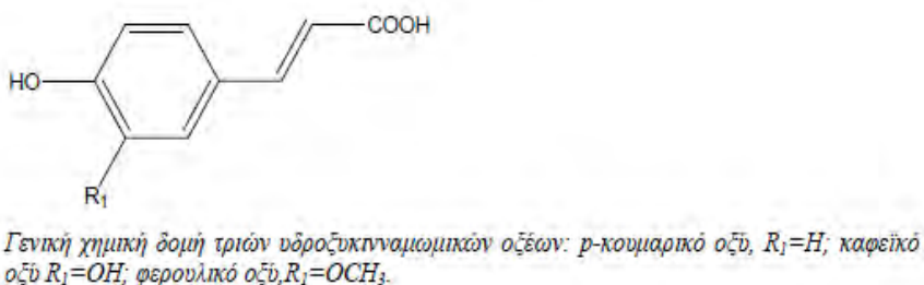
Εικόνα 11: Γενική δομή υδροξυκιναμικών οξέων.
