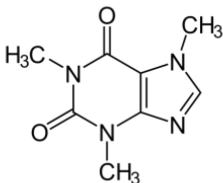
Εικόνα 14: Δομή καφεΐνης
