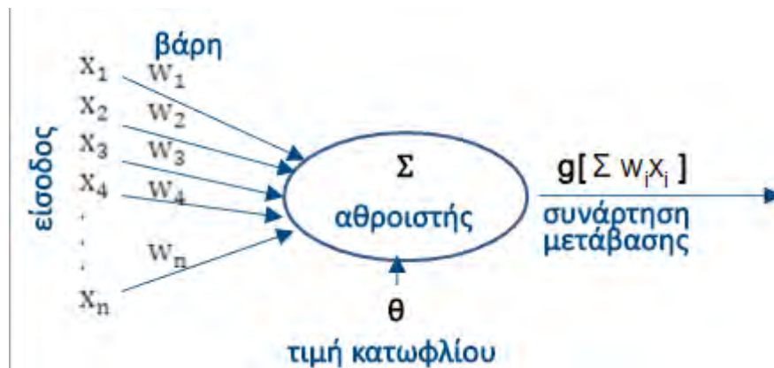
Εικόνα 4.1.1: Δομή και λειτουργία ενός νευρώνα
