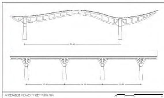
ΑΚΟΣΙΑΣΤΙΣ ΠΕΛΑΞΕΥΣ ΥΠΟΣΤΥΛΩΜΑΤΩΝ
