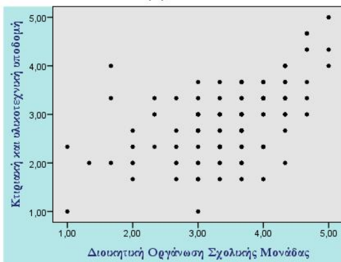
Διάγραμμα Σκεδασμού Ι Μεταβλητών Επαγγελματικής Ικανοποίησης Εκπαιδευτικών
