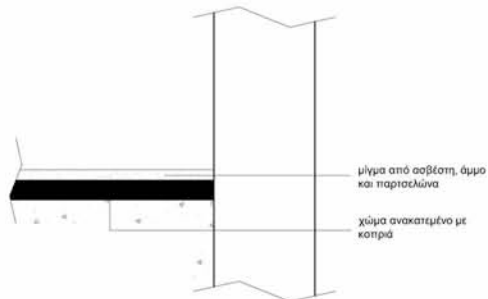
ΛΕΠΤΟΜΕΡΕΙΑ ΠΑΤΩΜΑΤΟΣ ΙΣΟΕΙΟΥ
