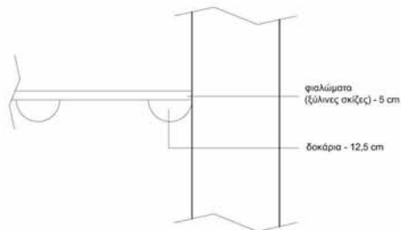
ΛΕΠΤΟΜΕΡΕΙΑ ΠΑΤΩΜΑΤΟΣ ΟΝΤΑ
