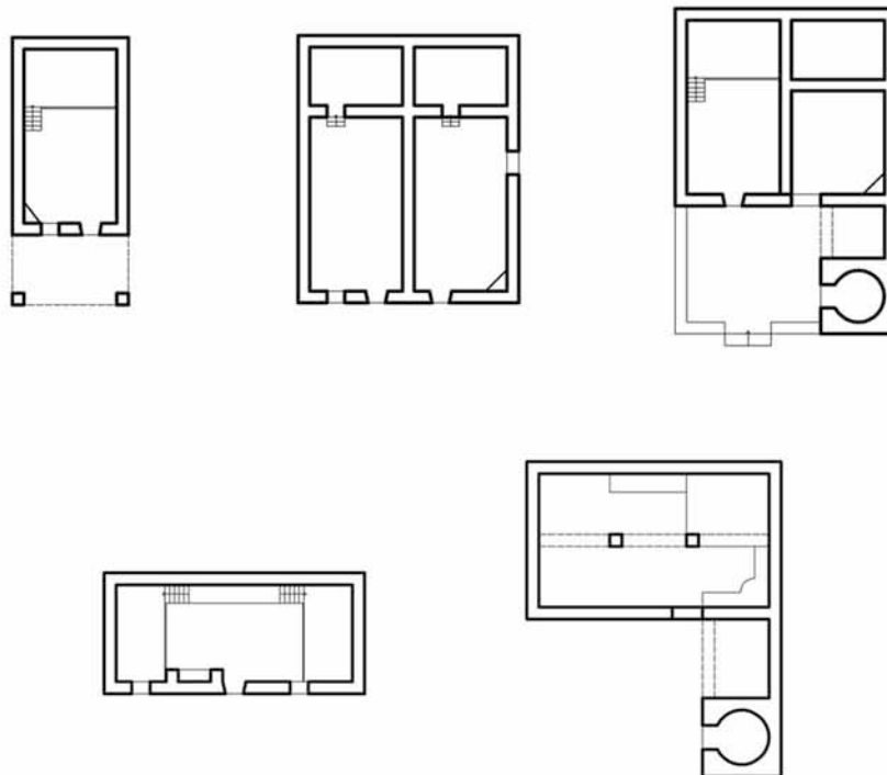
Τυπολογίες κατοικιών α) Θολιαστού σπιτιού β) σπιτιού με δώμα στενομέτρωπου ή πλατυμέτρωπου
