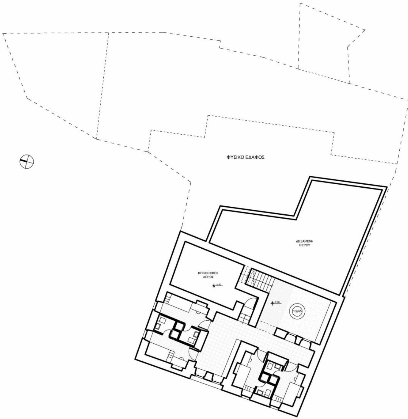
Κάτοψη υπογείου κλ. 1:200
