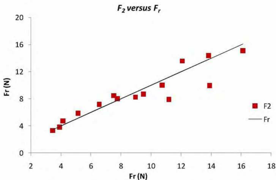
Σχήμα 4.10: Η δύναμη απώθησης του εργαλείου υπολογισμένη μέσω των προσαρμοσμένων θεωρητικών σχέσεων F_2 ως προς τις πειραματικές μετρήσεις F_r .
