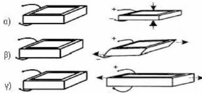
Σχήμα 6.9: Ο πιεζοηλεκτρικός κρύσταλλος εμφανίζει στην επιφάνειά του ηλεκτρικά φορτία αναλόγως την παραμόρφωσή του: α) Συμπίεση, β) Διάτμηση, γ) Εφελκυσμός.
