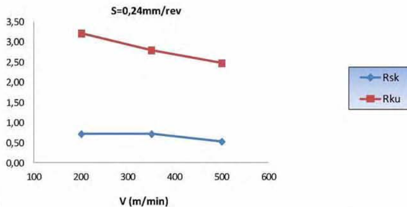
Σχήμα 7.10: Οι στατιστικές παράμετροι τραχύτητας συναρτήσει της ταχύτητας κοπής V , για κάθε πρόωση S α) S=0,05\text{mm/rev} , β) S=0,10\text{mm/rev} , γ) S=0,16\text{mm/rev} , δ) S=0,20\text{mm/rev} , ε) S=0,24\text{mm/rev} .
