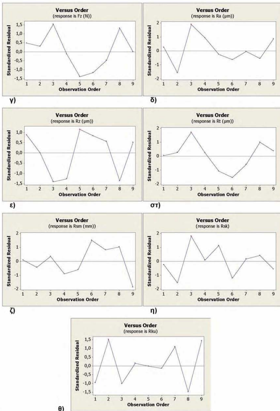
Σχήμα 8.15 (συνέχεια): Διαγράμματα των κανονικοποιημένων καταλοίπων των αποκρίσεων ως προς τη σειρά παρατήρησης: γ)Αξονική δύναμη F_z (N), δ)Μέση αριθμητική τραχύτητα R_a , ε)Ύψος δέκα σημείων R_z ( \mu\text{m} ), στ)Μέγιστο ύψος R_t , ζ)Μέσο διάστημα κορυφών R_{sm} , η)Λοξότητα R_{sk} , θ)Κυρτότητα R_{ku} .
