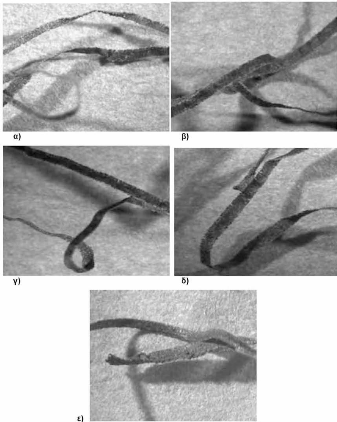
Σχήμα Δ.3: Η μορφολογία του αποβλίπτου για ταχύτητα κοπής V=200\text{m/min} , για κάθε πρόωση S α) S=0,05\text{mm/rev} : Συνεχές ταινιοειδές, β) S=0,10\text{mm/rev} : Συνεχές ταινιοειδές, γ) S=0,16\text{mm/rev} : Συνεχές ταινιοειδές, δ) S=0,20\text{mm/rev} : Ασυνεχές ταινιοειδές, ε) S=0,24\text{mm/rev} : Ασυνεχές ταινιοειδές.
