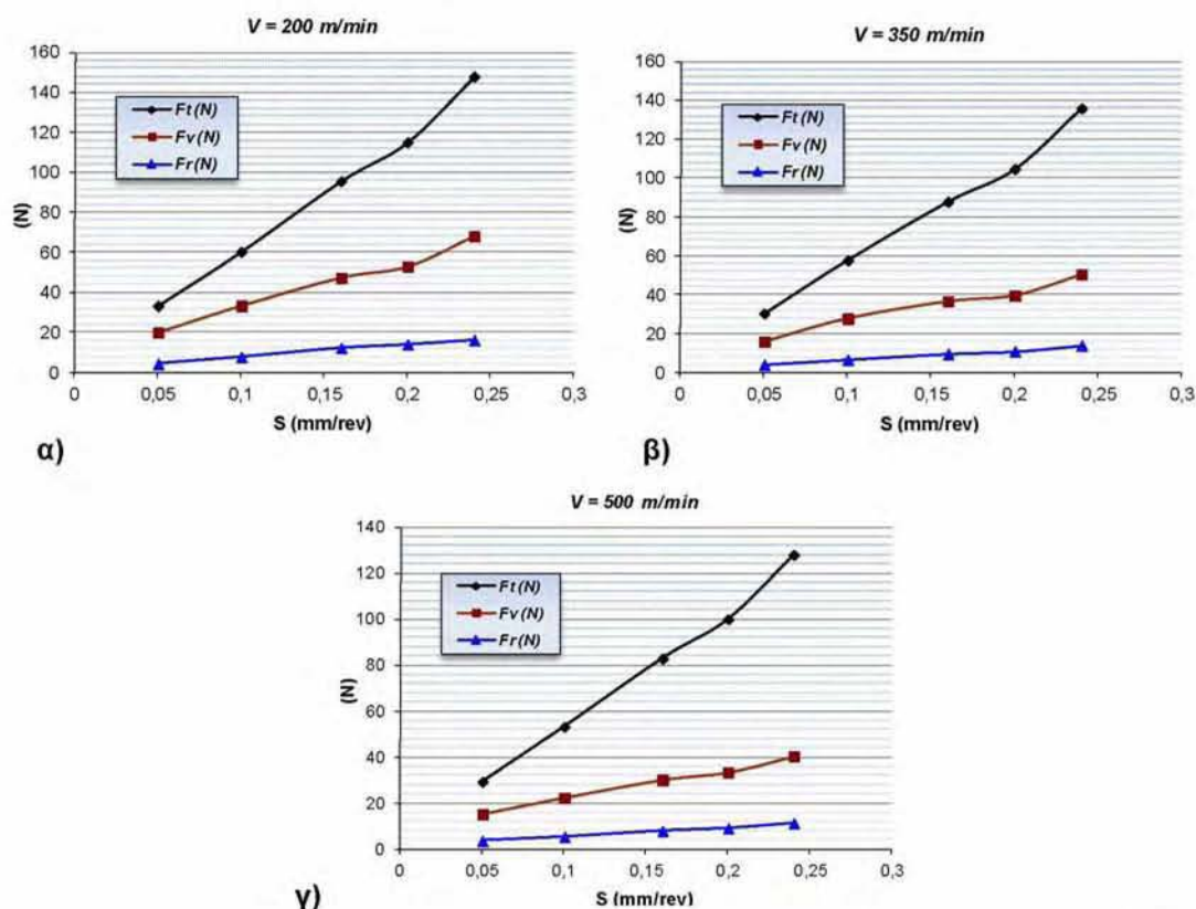
Σχήμα 7.4: Οι δυνάμεις κοπής συναρτήσει της πρόωσης S , για κάθε ταχύτητα κοπής V α) V=200 m/min, β) V=350 m/min, γ) V=500 m/min.
