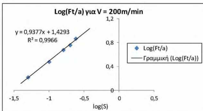
Σχήμα 4.11: Γραμμική συσχέτιση του \text{Log}(F_t/a) ως προς \text{Log}(s) για ταχύτητα κοπής 200m/min
