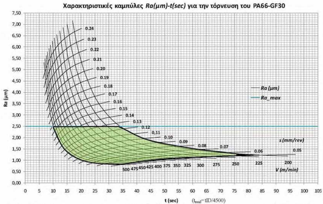
Σχήμα 7.33: Χαρακτηριστικές καμπύλες Ra(\mu m)-t(sec) για την τórνευση του PA66-GF30, επιλογή τιμών των παραγόντων βάσει περιορισμού στην τραχύτητα.
