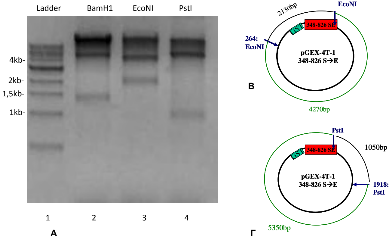
Εικόνα 18. Α) Έλεγχος του προσανατολισμού της ένθεσης του HIF-1\alpha^{348-826} S \rightarrow E στον pGEX-4T με πέψεις με EcoNI και PstI . Ηλεκτροφόρηση σε πηκτή αгарόζης 1%
