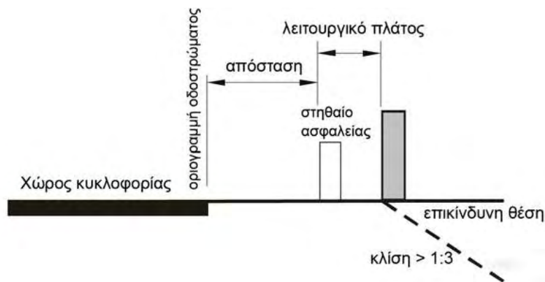
Διάταξη των μόνιμων στηθαίων ασφαλείας σε συνάρτηση με το λειτουργικό πλάτος και τον κυκλοφοριακό χώρο
