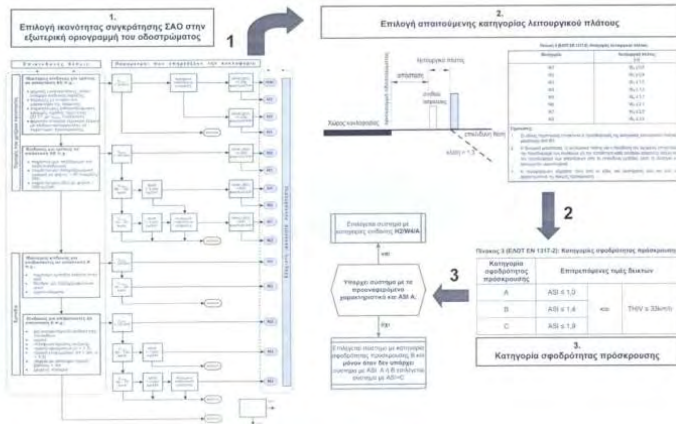
Επιλογή κατηγοριών επίδοσης μόνιμων στηθαίων ασφαλείας στην εξωτερική οριογραμμή οδοστρώματος
