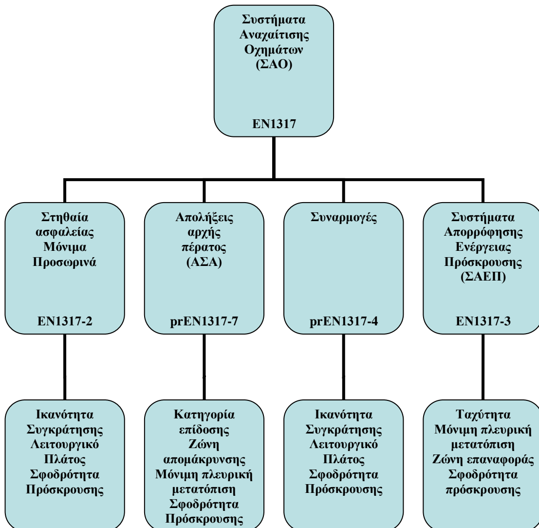
Καθορισμός κατηγοριών επίδοσης κατά ΕΛΟΤ EN1317
