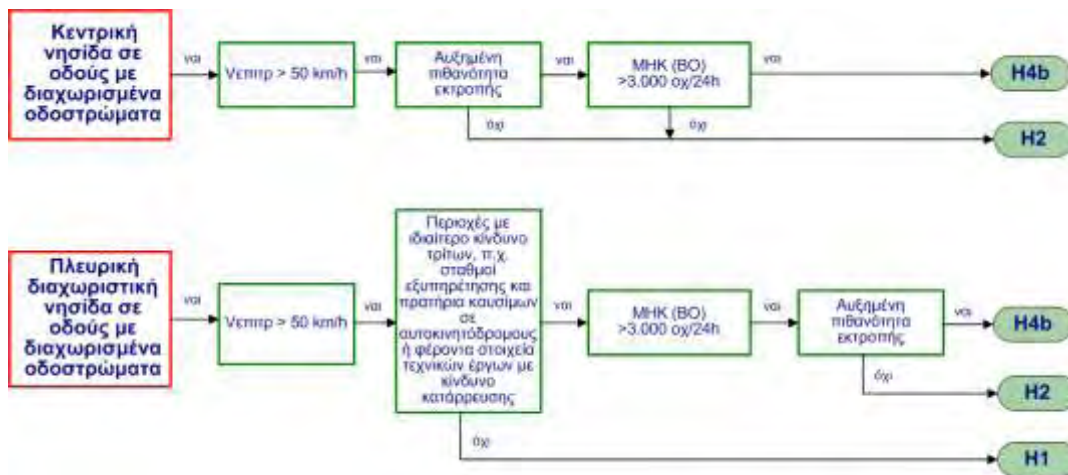
Κριτήρια εφαρμογής μόνιμων στηθαίων ασφαλείας σε κεντρικές & πλευρικές διαχ/κές νησίδες
