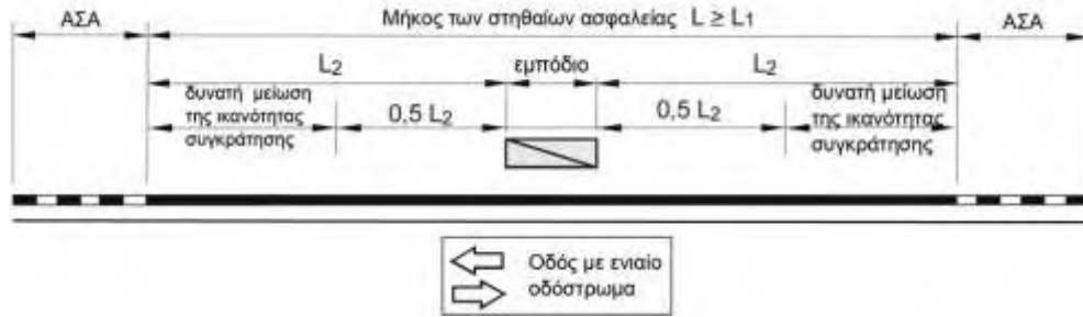
Μήκη στηθαίων ασφαλείας παράλληλα τοποθετημένα σε οδό με ενιαίο οδόστρωμα
