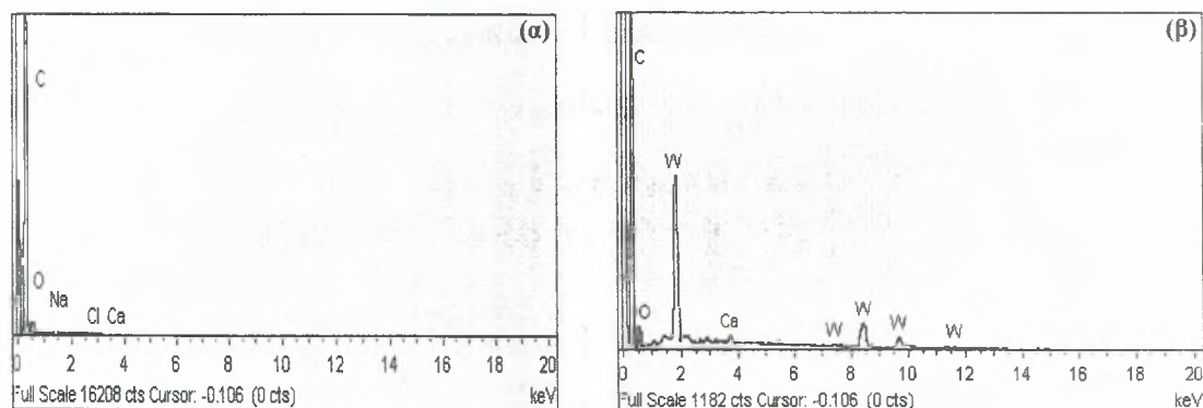
Σχήμα 5.4 Αναλύσεις φασματομετρίας διασποράς ενέργειας ακτίνων X (EDX) των δειγμάτων (α) CMSs και (β) TCMS, αντίστοιχα.
