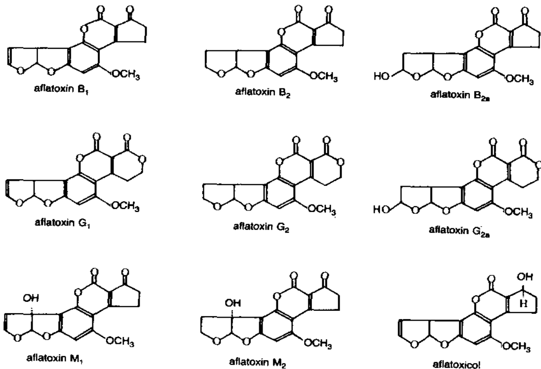
Εικόνα 2: Χημικοί τύποι των σημαντικότερων αφλατοξινών.
