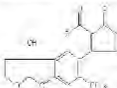
Χημική σύνθεση της Αflatoξίνης M1
