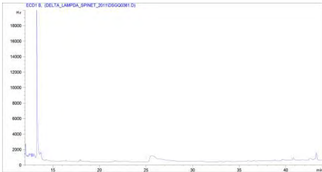
Εικόνα 11. Χρωματογράφημα εκχυλίσματος μάρτυρα για το υπόστρωμα ελαιόλαδο (βιολογικής παραγωγής ελαιόλαδο).
