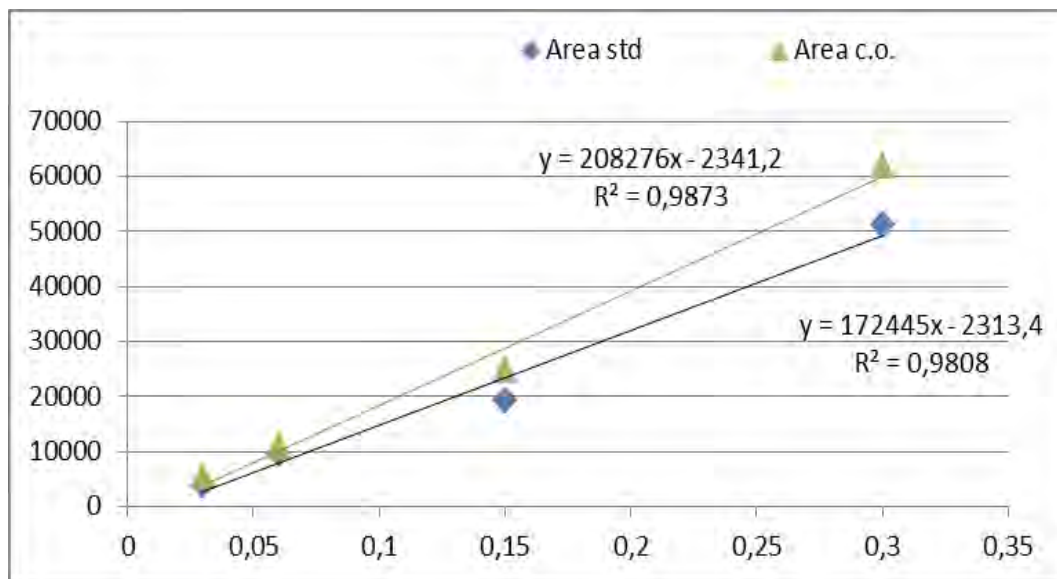
Διάγραμμα 6. Καμπύλη βαθμονόμησης για τη δραστική ουσία Cypermethrin σε εκχύλιση υποστρώματος καλαμποκέλαιου
