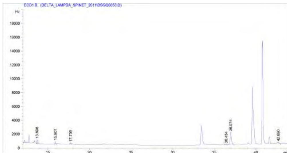
Εικόνα 18. Χρωματογράφημα εκχυλίσματος δείγματος εμπορικού μίγματος ελαίων (κραμβέλαιο, αραβοσιτέλαιο και ηλιέλαιο) –Α.
