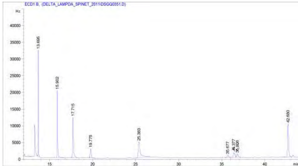
Εικόνα 16. Χρωματογράφημα μίγματος προτύπου διαλύματος των φυτοπροστατευτικών ουσιών – στόχων συγκέντρωσης 0,3mg/L για κάθε δραστική ουσία, σε υπόστρωμα ελαιολάδου.
