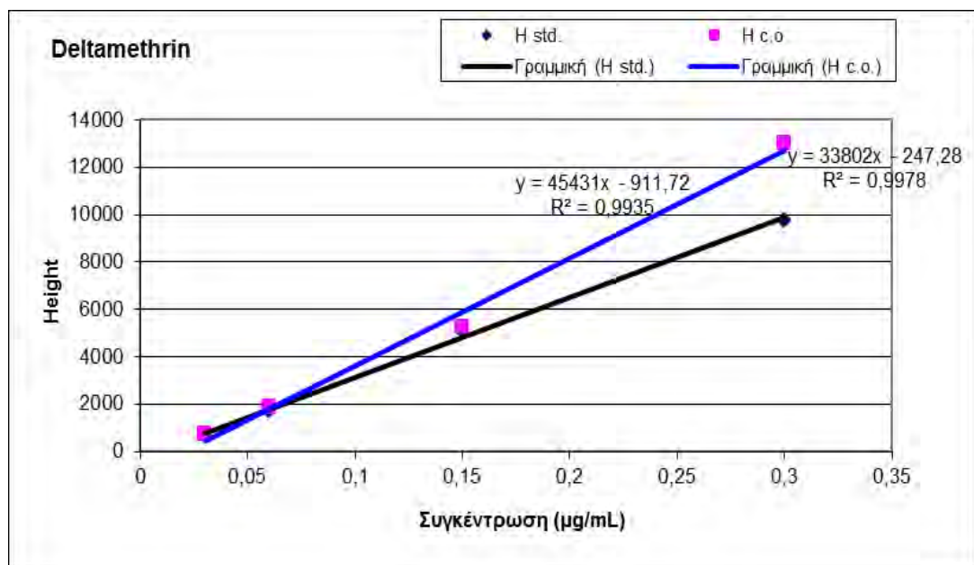
Διάγραμμα 7. Καμπύλη βαθμονόμησης για τη δραστική ουσία Deltamethrin σε εκχύλιση υποστρώματος καλαμποκέλαιου
