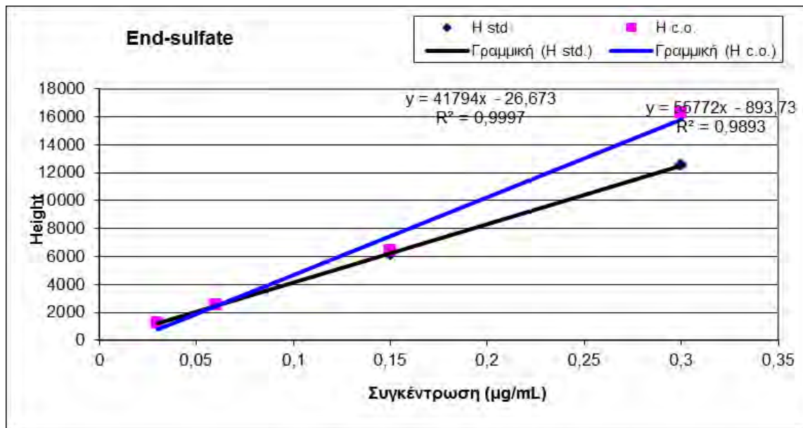
Διάγραμμα 3. Καμπύλη βαθμονόμησης για τη δραστική ουσία Endosulfan sulfate σε εκχύλισμα υποστρώματος καλαμποκέλαιου
