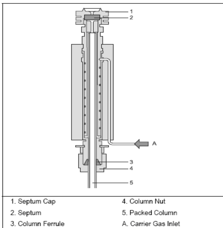
Σχήμα 3.14. Packed Column Injector (PCI)
