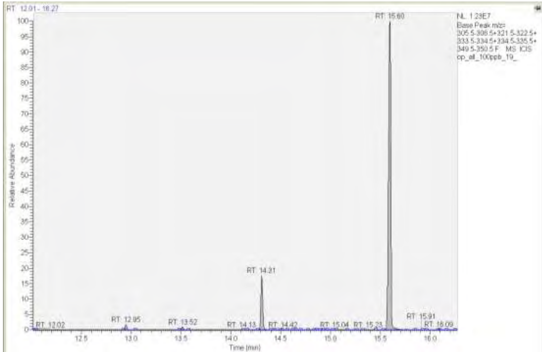
Φάσμα GC 4.3. Ανάλυση διαλύματος όλων των μεταβολιτών με DBP ως I.S. σε συγκέντρωση 100ppb. (base peak)
