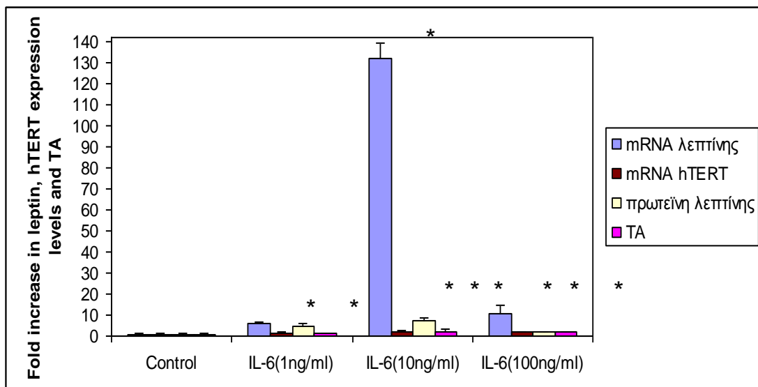
Διάγραμμα 20. Επίδραση της IL-6 στα επίπεδα έκφρασης της λεπτίνης (mRNA και πρωτεΐνης) και της hTERT (mRNA και TA) στα HepG2 κύτταρα. Τα ραβδογράμματα παρουσιάζουν τη μέση τιμή και την τυπική απόκλιση από τρία ανεξάρτητα πειράματα που αξιολογήθηκαν εις τριπλούν το καθένα. Οι αστερίσκοι (*) επισημαίνουν τα επίπεδα στατιστικής σημασίας ( p < 0.001 για τη λεπτίνη και p < 0.05 για την hTERT) των διαφορών των συνθηκών από την συνθήκη ελέγχου (control).
