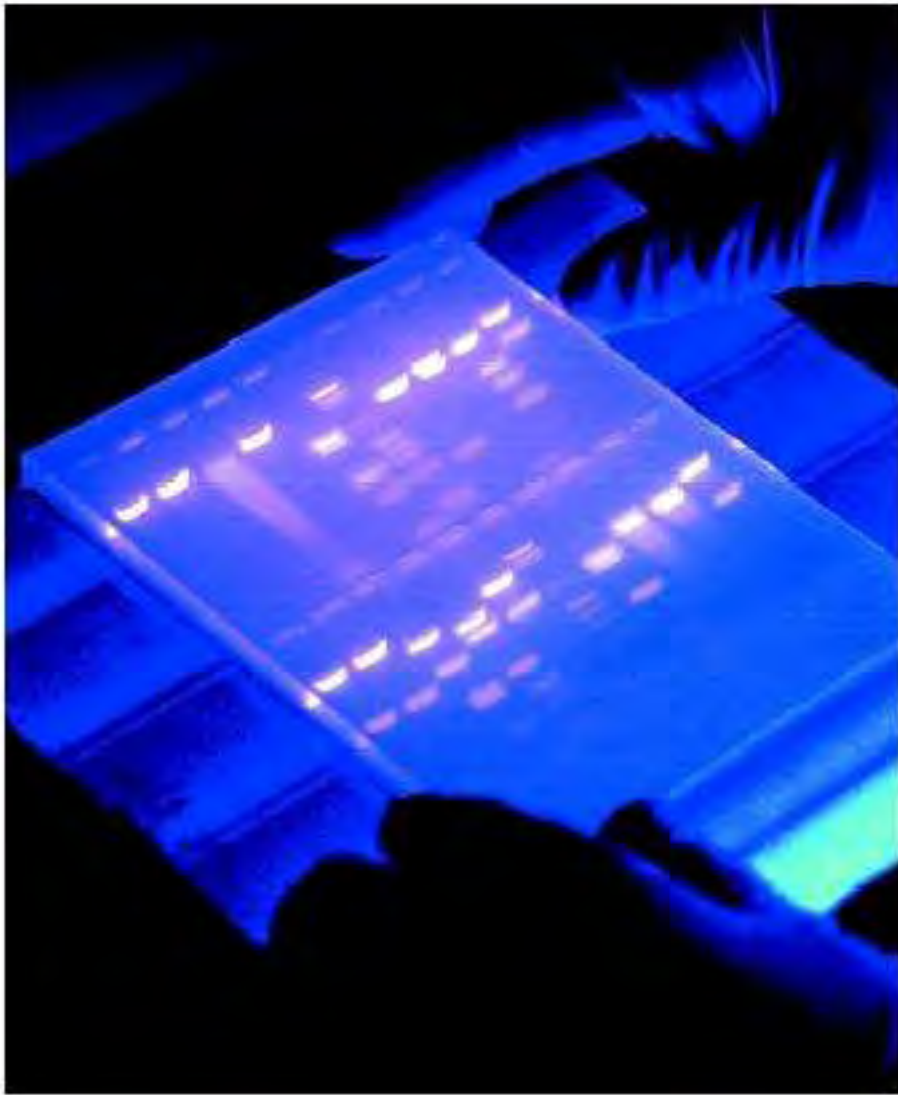
Εικόνα 12. Gel ηλεκτροφόρησης
