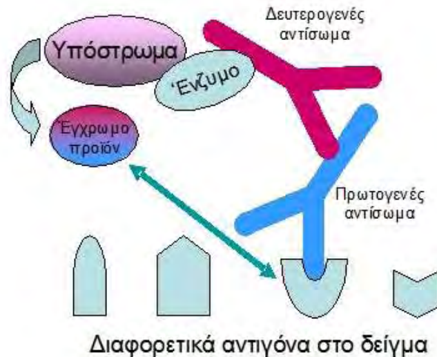
Εικόνα 6. Μέθοδος ELISA
