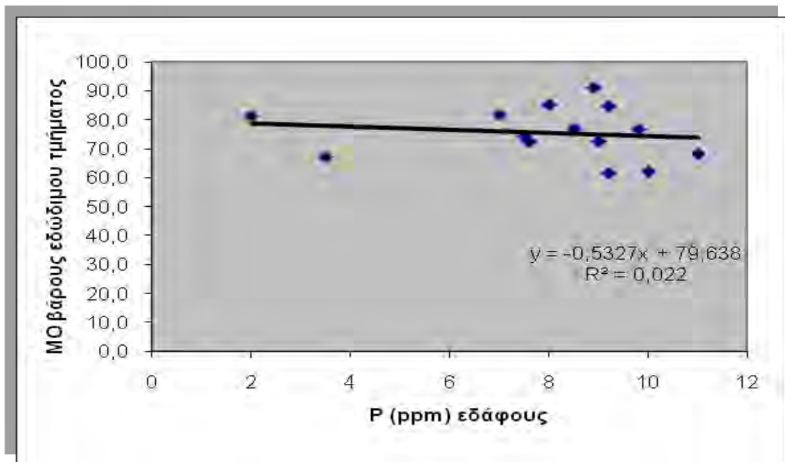
Διάγραμμα 68. Η συγκέντρωση P στο έδαφος σε βάθος 0-30 cm σε συνάρτηση με τον μέσο όρο του βάρους του εδώδιμου τμήματος των καρπών της πορτοκαλιάς
