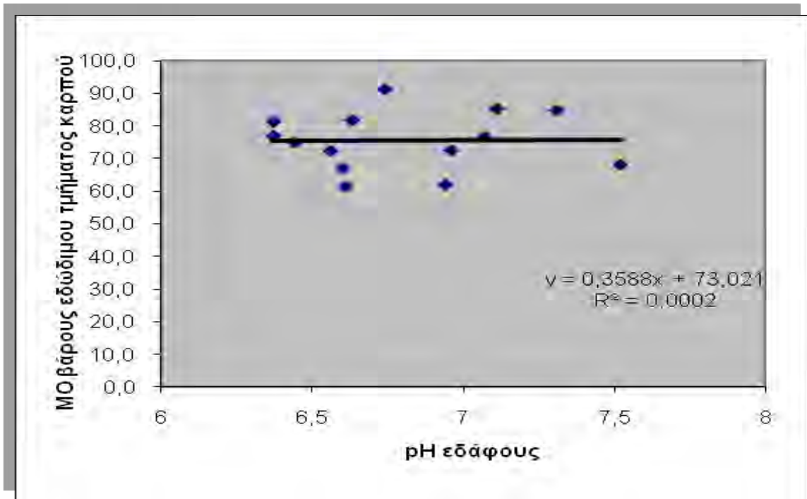
Διάγραμμα 9. Το pH του εδάφους σε σχέση με τον μέσο όρο του βάρους του εδώδιμου τμήματος του καρπού της πορτοκαλιάς
