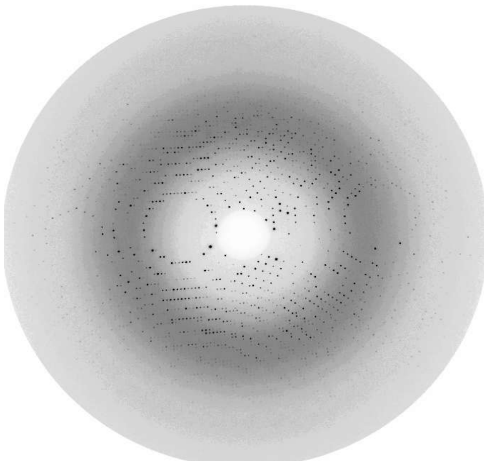
Εικόνα 17 : παράδειγμα περιθλασιγράμματος. Το συγκεκριμένο περιθλασίγραμμα προέκυψε από περίθλαση ακτίνων X κρυστάλλου της φωσφορυλάσης του γλυκογόνου εμποτισμένου με έναν αναστολέα του ενζύμου.
