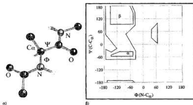
Εικόνα 23: α) Ορισμός των \phi (C \alpha -N) και \psi (C \alpha -C) διεδρων γωνιών και β) το διάγραμμα Ramachandran για κατάλοιπα εκτός γλυκίνης (περιοχή χωρίς γράμμα) ενώ η περιοχή \alpha : δεξιόστροφη \alpha -έλικα και η περιοχή \beta : αντιπαράλληλη-παράλληλη πτυχωτή επιφάνεια [Rhodes].
