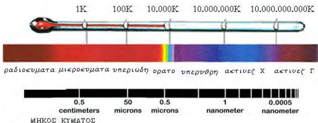
Εικόνα 14: Το ηλεκτρομαγνητικό φάσμα.
