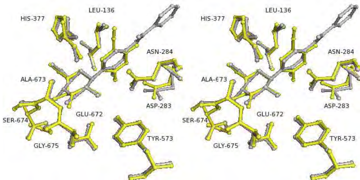
Εικόνα 42: Υπέρθηση του συμπλόκου GPb-DK12 πάνω στο σύμπλοκο GPb-DK2. Με κίτρινο χρώμα φαίνεται το σύμπλοκο GPb-DK12, ενώ με γκρι το σύμπλοκο GPb-DK2
