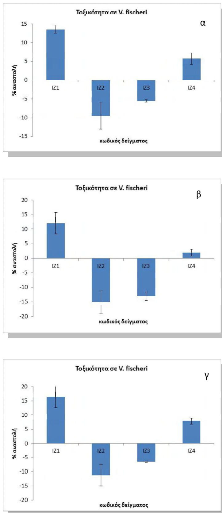
Διάγραμμα 4.1: Τοξικότητα των υγρών έκπλυσης στο V. fischeri α) για χρόνο μέτρησης 5 min, β) για χρόνο μέτρησης 15 min γ) για χρόνο μέτρησης 30 min
