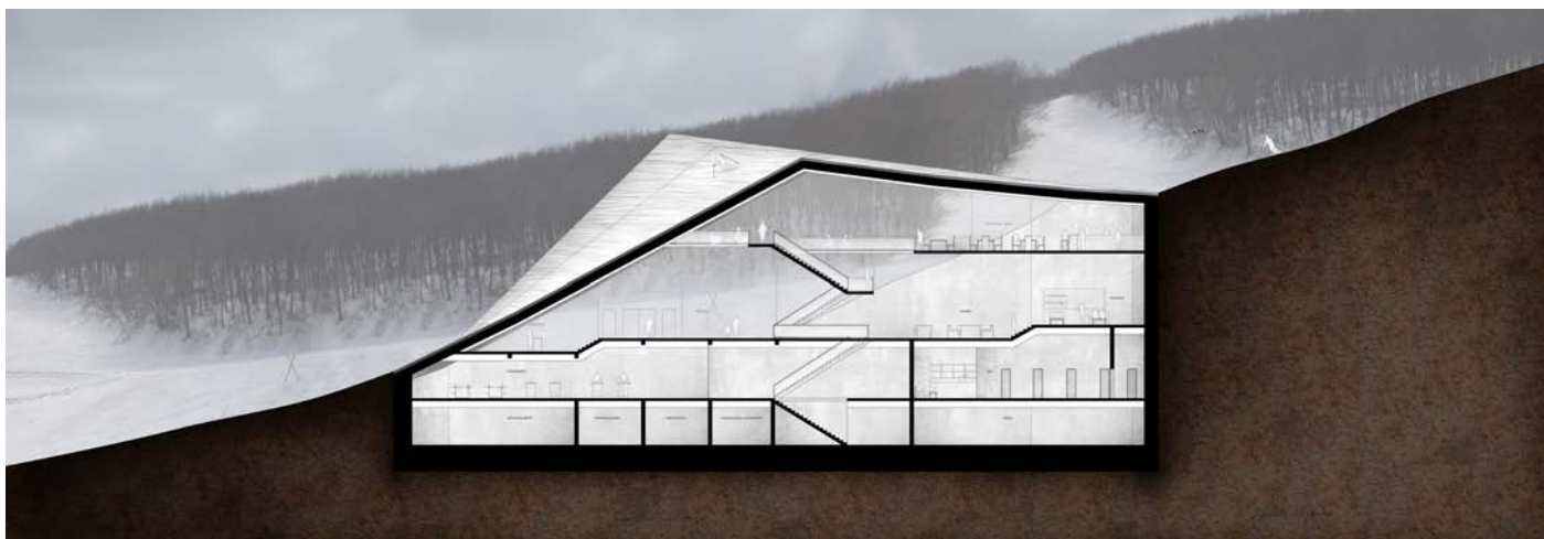
Τομή B-B'
