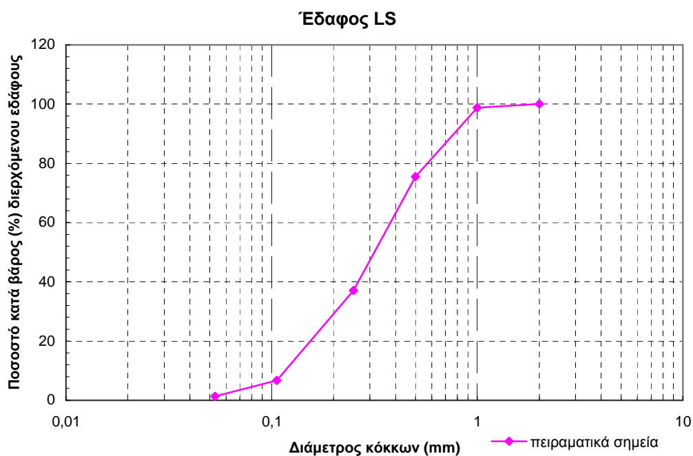
Σχήμα 3.2.β. Κοκκομετρική καμπύλη εδαφικού δείγματος LS
