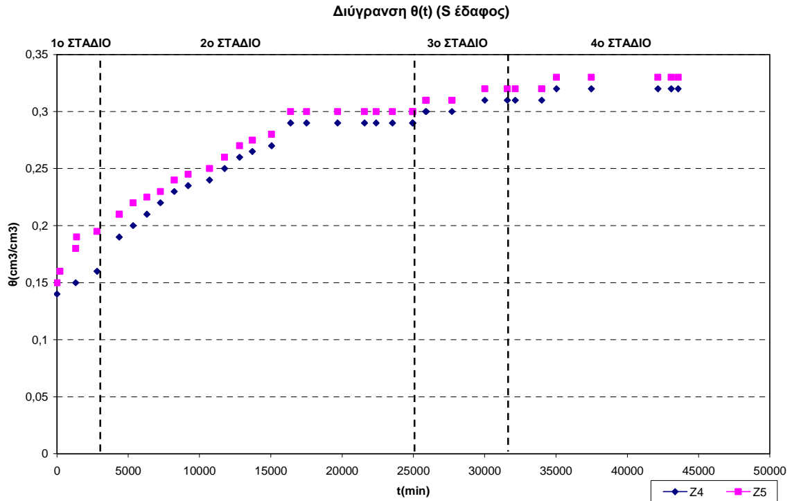
Σχήμα 3.20: Πειραματικές τιμές της υγρασίας ως προς το χρόνο στο αμμώδες έδαφος (κάτω στρώση), κατά τη 2 η διύγρανση
