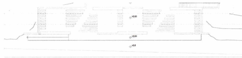
απόσπασμα 5 - διαμόρφωση κατά μήκος του τείχους κλίμακα 1 : 100
