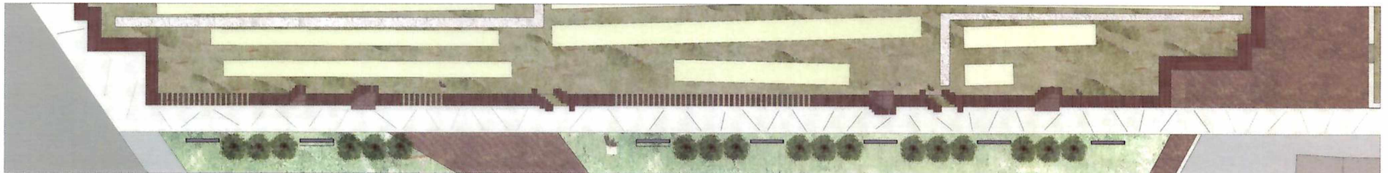
απόσπασμα 3-νεκροταφείο Ευαγγελίστριας κάτωψη ανατολικής περιφέρειας κλίμα: 1 : 250
