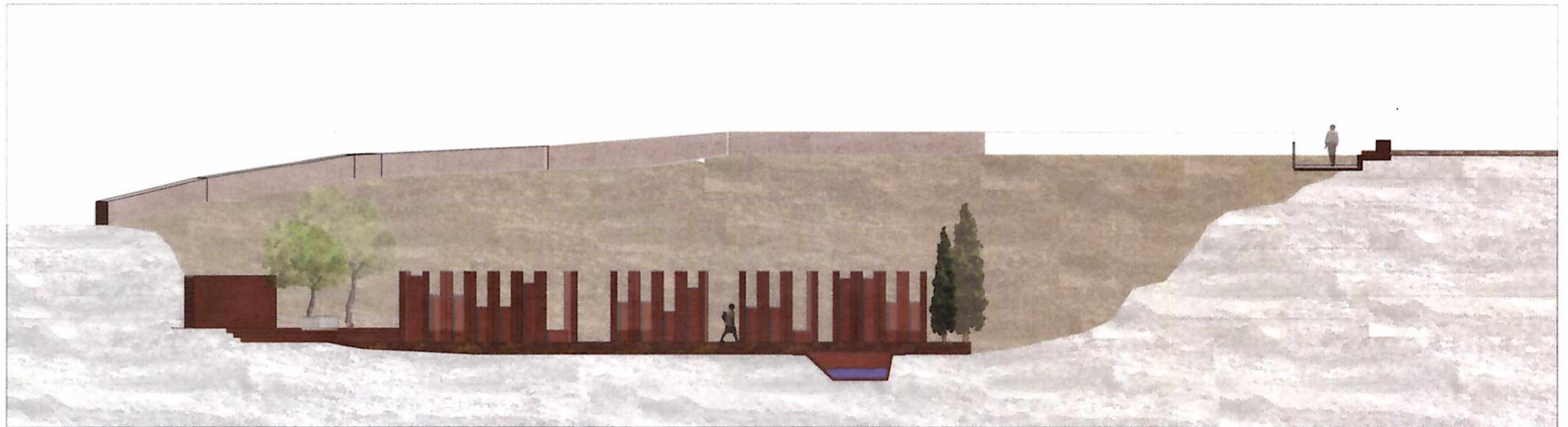
απόσπασμα 7 - στάση χαμηλό δίπλα στο ρέμα λιπαστή κλίμακ. 1 : 100
