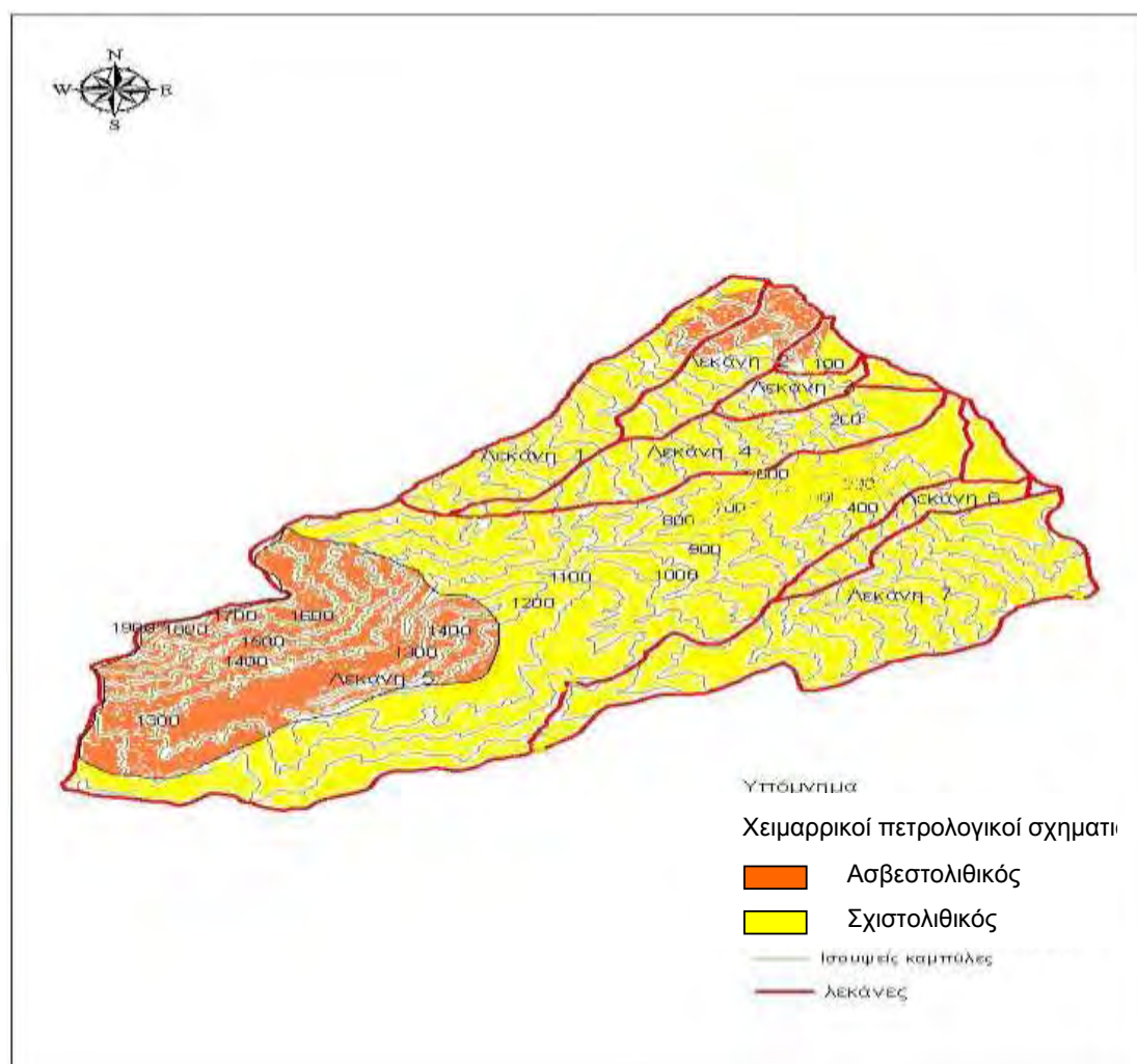
Εικόνα 13 : Χειμαρρικοί πετρωολογικοί σχηματισμοί στη περιοχή έρευνας.
