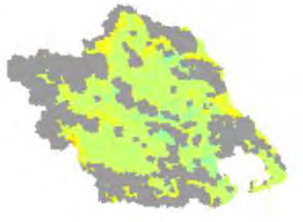
Χάρτης TVDI 2004_4_3
