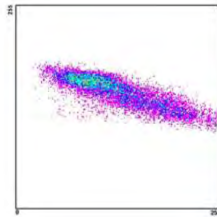
Διάγραμμα διασποράς 2005_6_3
