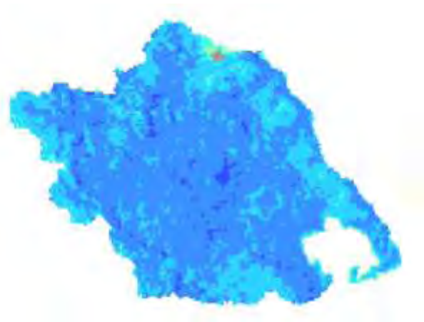
Χάρτης TVDI 2004_7_3
