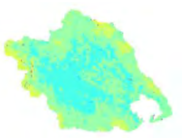
Χάρτης TVDI 2001_9_3
