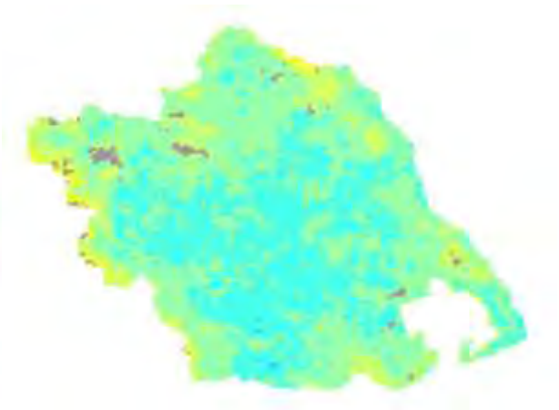
Χάρτης TVDI 2002_10_3
