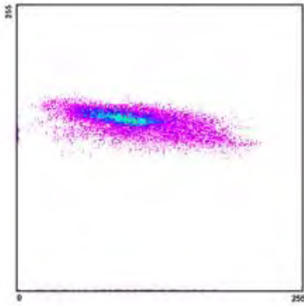
Διάγραμμα διασποράς 2005_9_4
