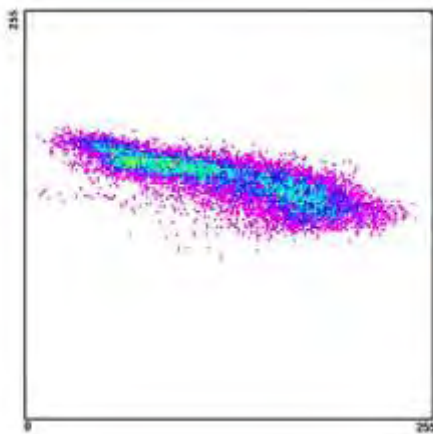
Διάγραμμα διασποράς 2005_10_4
