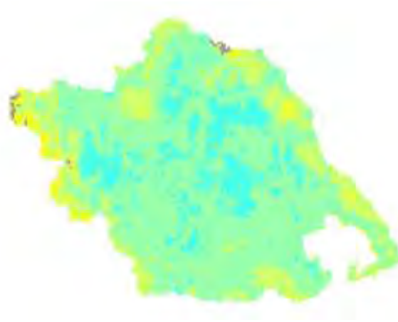
Χάρτης TVDI 2001_4_3
