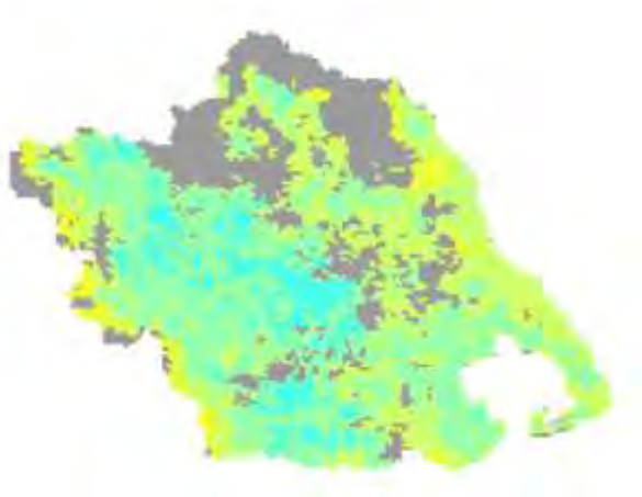
Χάρτης TVDI 2001_5_1
