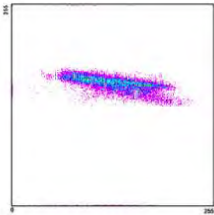
Διάγραμμα διασποράς 2001_7_3
