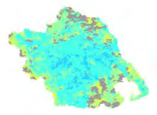
Χάρτης TVDI 2002_9_4
