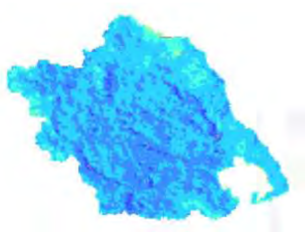
Χάρτης TVDI 2005_8_4
