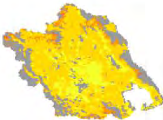
Χάρτης TVDI 2001_1_5
