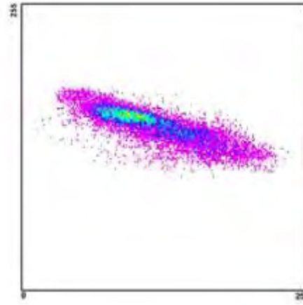
Διάγραμμα διασποράς 2004_10_1
