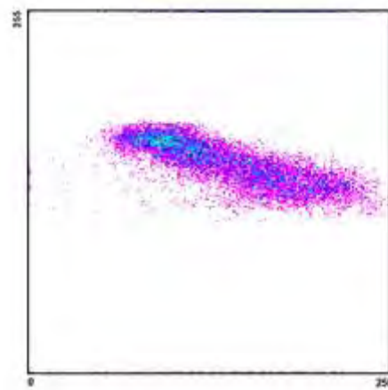
Διάγραμμα διασποράς 2005_6_1
