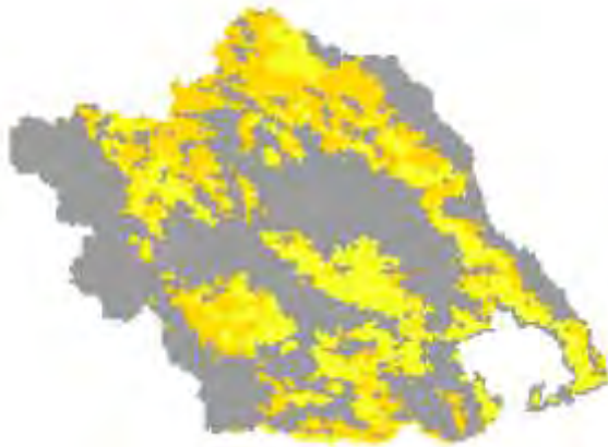
Χάρτης TVDI 2001_1_1
