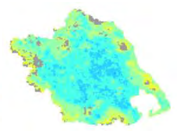
Χάρτης TVDI 2002_4_1
