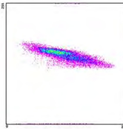
Διάγραμμα διασποράς 2003_9_5
