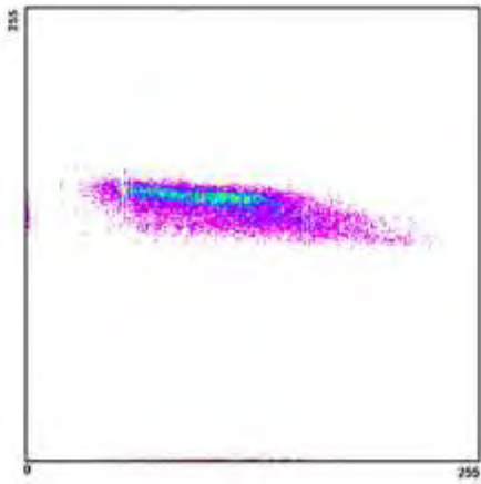
Διάγραμμα διασποράς 2001_7_1
