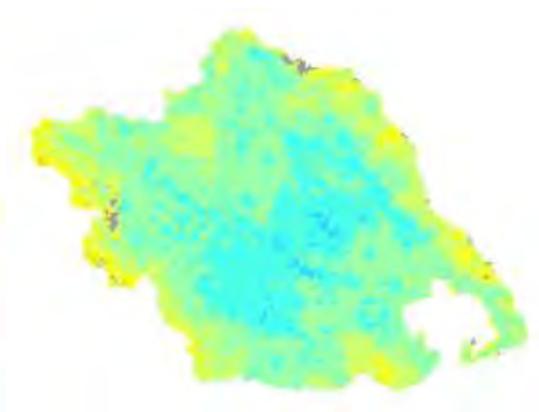
Χάρτης TVDI 2001_3_2
