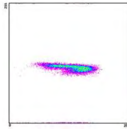
Διάγραμμα διασποράς 2002_11_2
