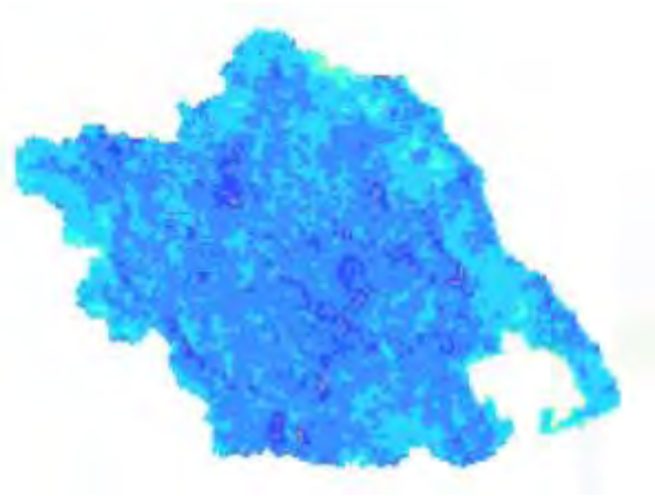
Χάρτης TVDI 2005_8_2
