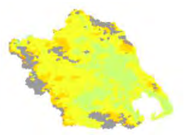
Χάρτης TVDI 2002_11_1
