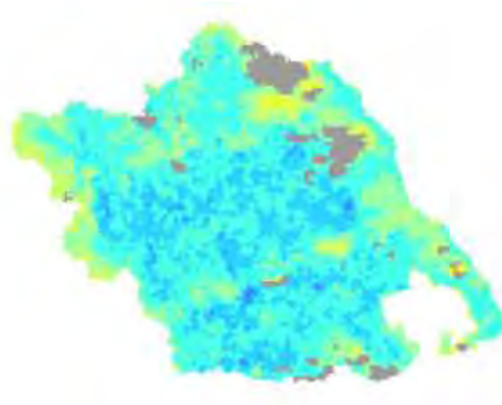
Χάρτης TVDI 2004_5_4
