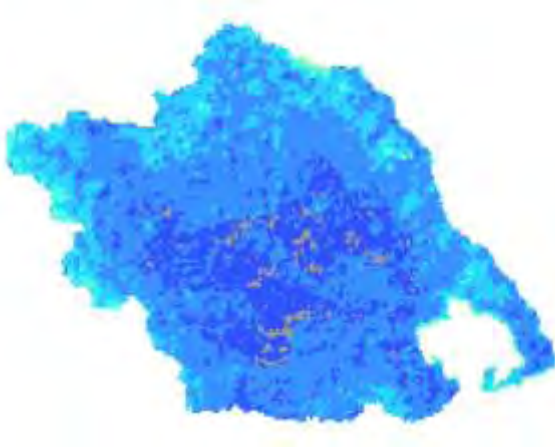
Χάρτης TVDI 2002_8_2
