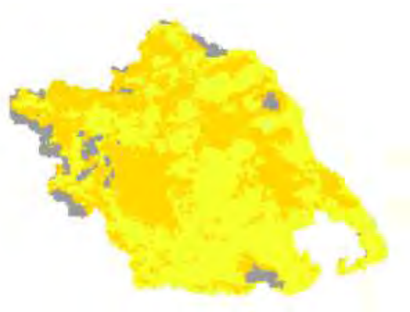
Χάρτης TVDI 2005_1_2
