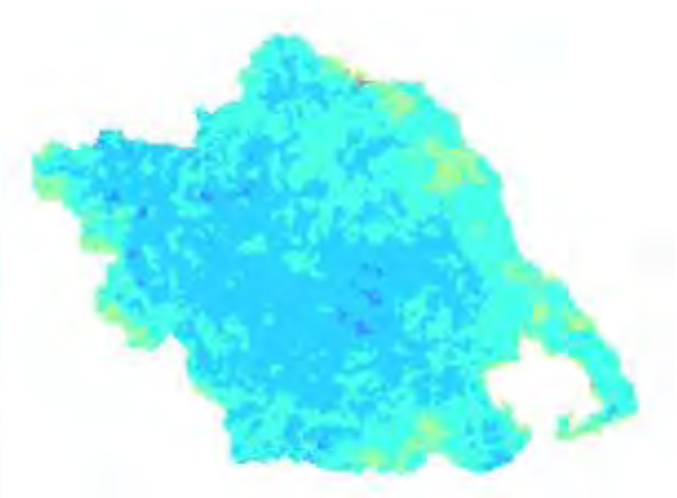
Χάρτης TVDI 2004_9_3
