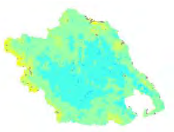
Χάρτης TVDI 2001_9_1
