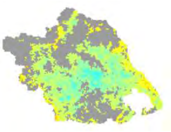
Χάρτης TVDI 2001_4_2
