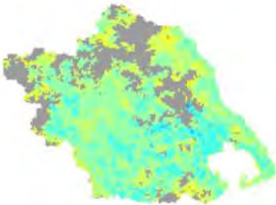
Χάρτης TVDI 2002_4_4
