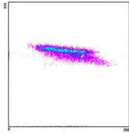
Διάγραμμα διασποράς 2001_7_2
