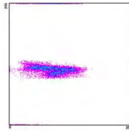
Διάγραμμα διασποράς 2002_11_4
