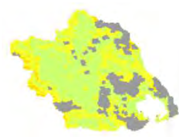
Χάρτης TVDI 2003_11_2
