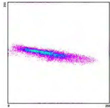
Διάγραμμα διασποράς 2005_10_3
