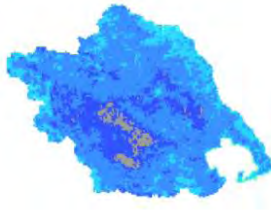
Χάρτης TVDI 2002_8_1
