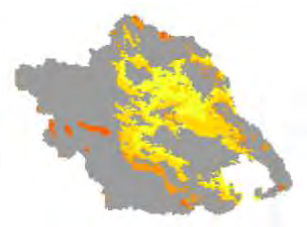
Χάρτης TVDI 2002_12_2
