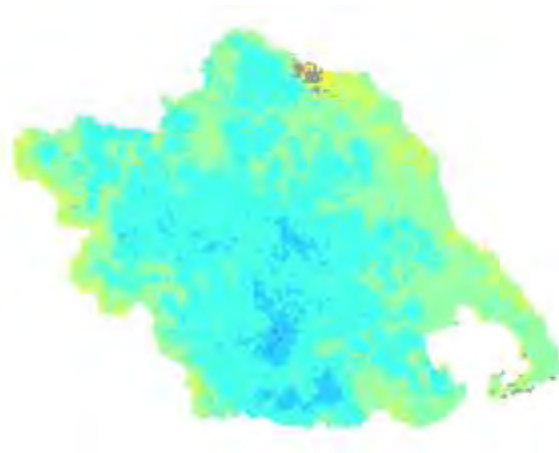
Χάρτης TVDI 2001_5_2
