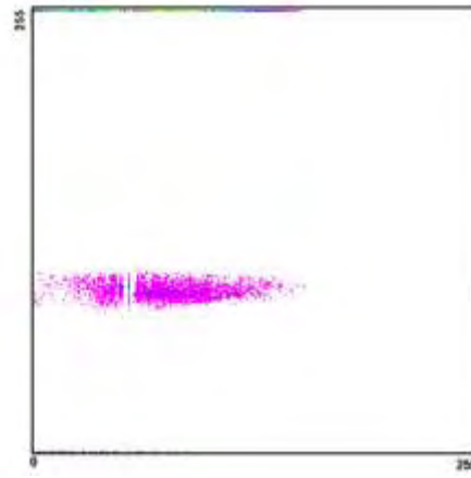
Διάγραμμα διασποράς 2002_10_3
