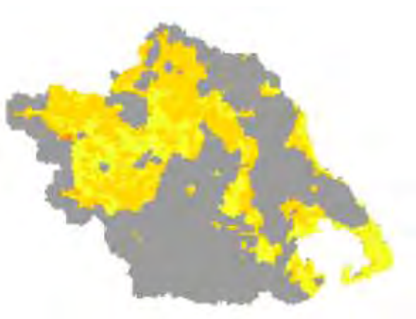
Χάρτης TVDI 2005_1_3
