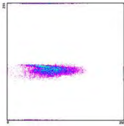
Διάγραμμα διασποράς 2002_11_1
