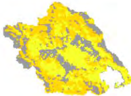
Χάρτης TVDI 2001_1_2
