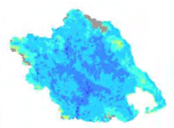
Χάρτης TVDI 2005_6_2
