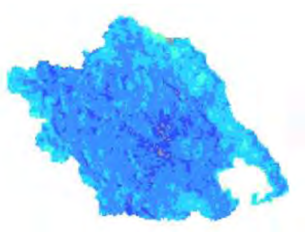
Χάρτης TVDI 2004_8_2
