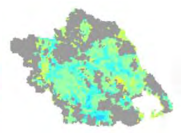
Χάρτης TVDI 2005_5_5
