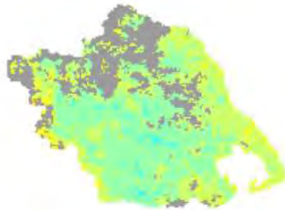
Χάρτης TVDI 2002_4_3
