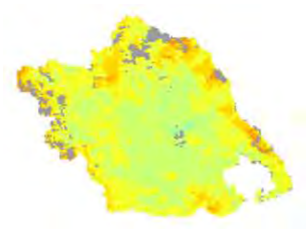
Χάρτης TVDI 2001_3_1
