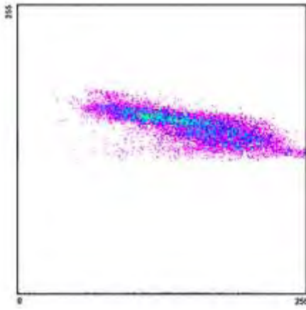
Διάγραμμα διασποράς 2005_5_2
