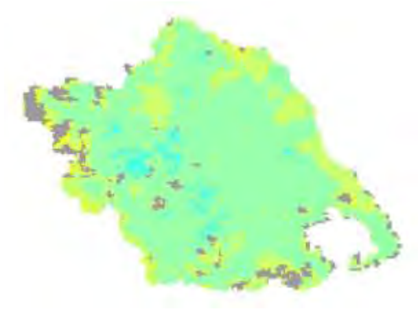
Χάρτης TVDI 2001_5_3
