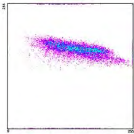
Διάγραμμα διασποράς 2003_7_4
