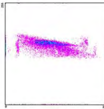
Διάγραμμα διασποράς 2003_9_3
