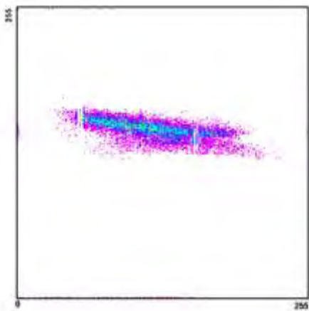
Διάγραμμα διασποράς 2001_7_5
