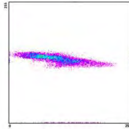
Διάγραμμα διασποράς 2004_10_3
