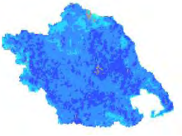
Χάρτης TVDI 2002_7_3
