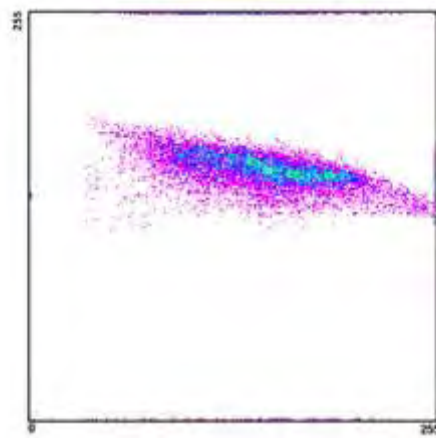
Διάγραμμα διασποράς 2003_8_1
