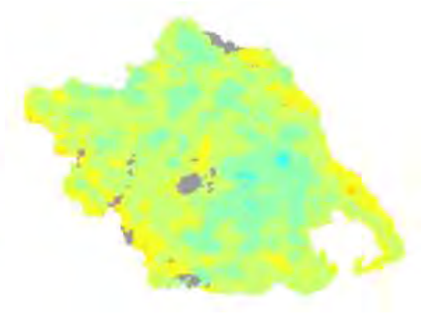
Χάρτης TVDI 2002_3_1
