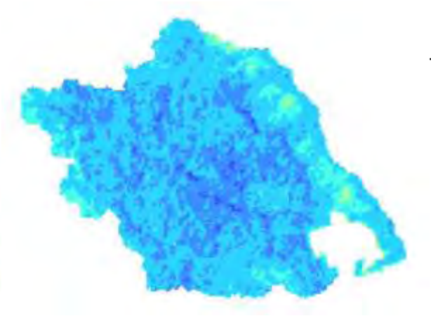
Χάρτης TVDI 2004_8_4
