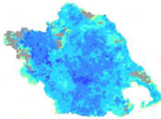
Χάρτης TVDI 2002_5_4
