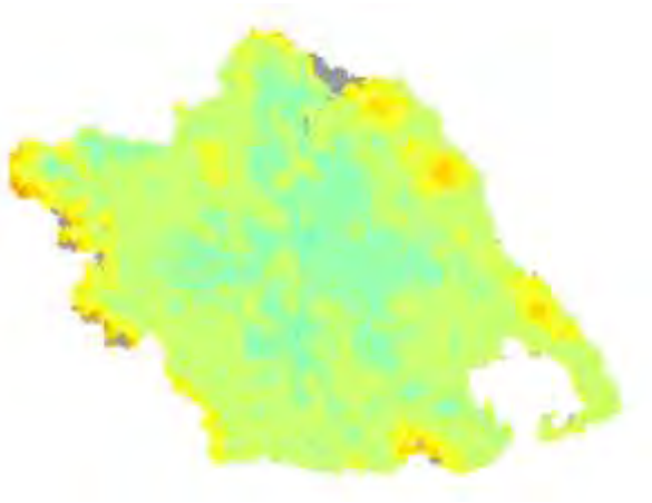
Χάρτης TVDI 2001_4_4
