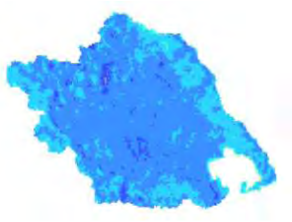
Χάρτης TVDI 2004_7_1
