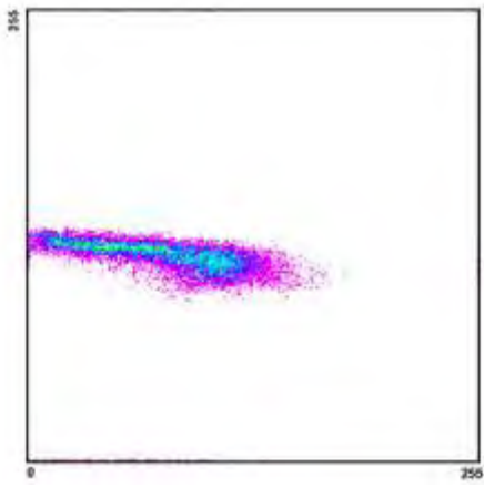
Διάγραμμα διασποράς 2005_11_1
