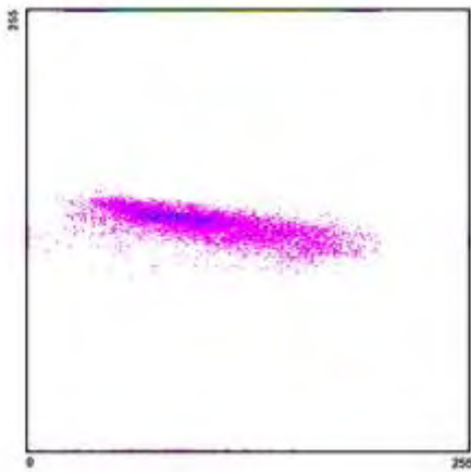
Διάγραμμα διασποράς 2005_10_2
