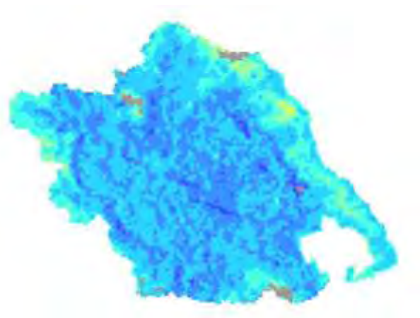
Χάρτης TVDI 2005_9_1
