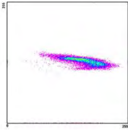
Διάγραμμα διασποράς 2002_10_2
