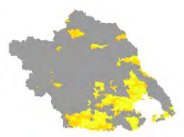
Χάρτης TVDI 2002_12_4
