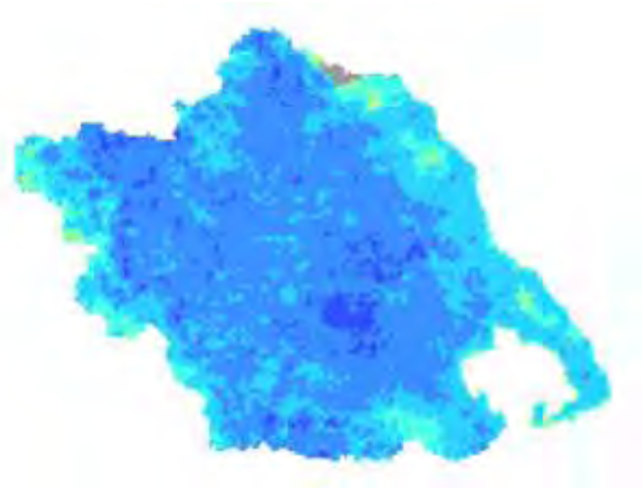
Χάρτης TVDI 2003_5_2
