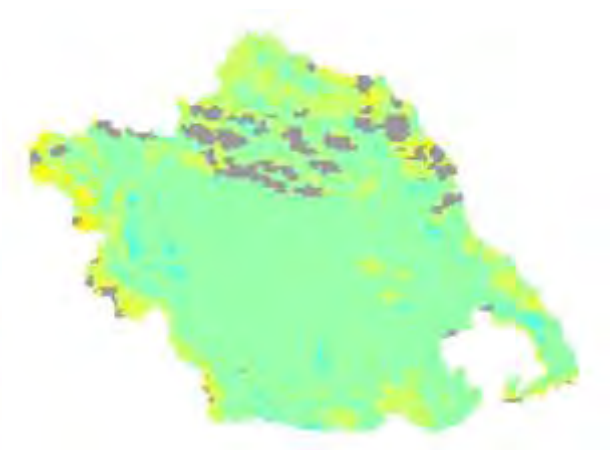
Χάρτης TVDI 2003_10_3
