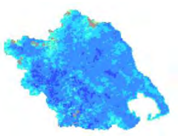
Χάρτης TVDI 2003_6_2
