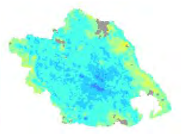
Χάρτης TVDI 2004_9_1
