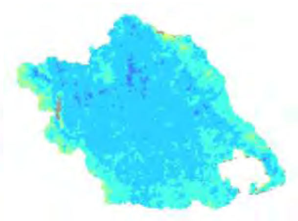
Χάρτης TVDI 2001_6_2
