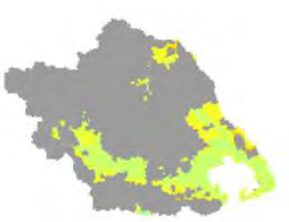
Χάρτης TVDI 2003_1_2
