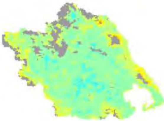
Χάρτης TVDI 2002_4_2
