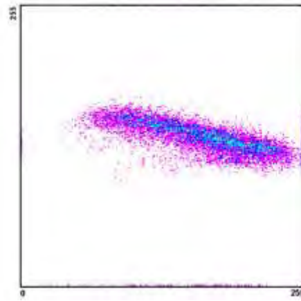
Διάγραμμα διασποράς 2004_5_4
