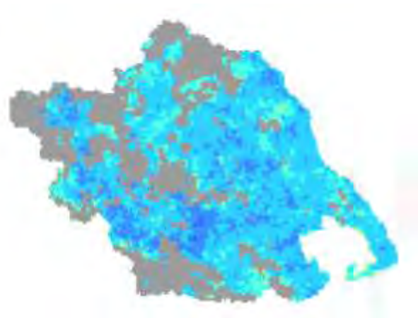
Χάρτης TVDI 2003_5_4
