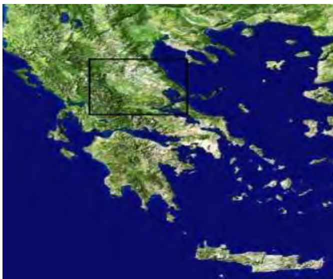
Εικόνα 2.5: Χάρτης βλάστησης της περιοχής της Θεσσαλίας.
