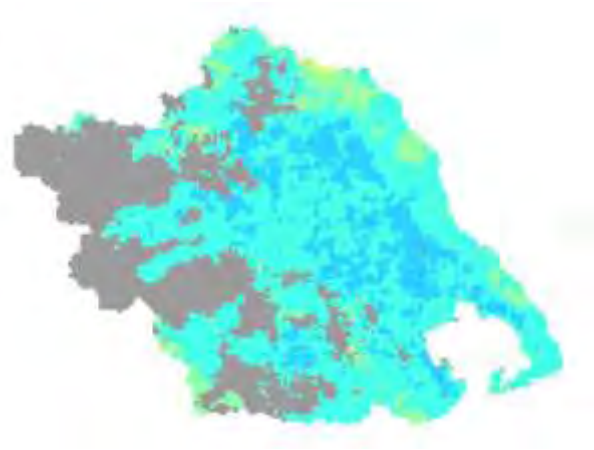
Χάρτης TVDI 2001_8_3
