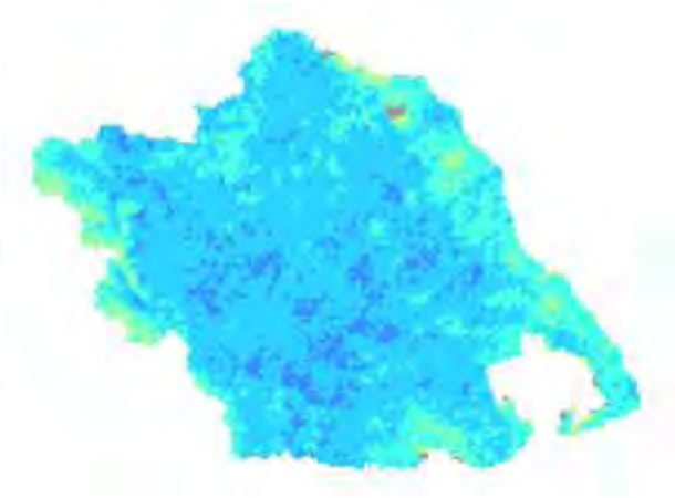
Χάρτης TVDI 2003_9_4
