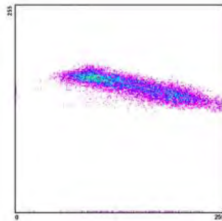
Διάγραμμα διασποράς 2004_6_3
