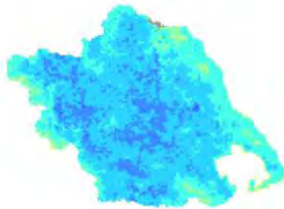
Χάρτης TVDI 2002_4_5
