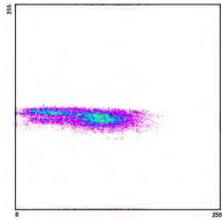
Διάγραμμα διασποράς 2005_11_2
