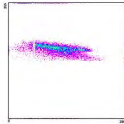
Διάγραμμα διασποράς 2001_7_4
