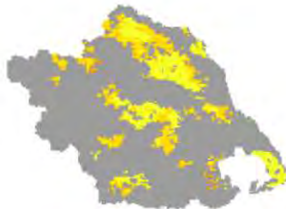
Χάρτης TVDI 2001_1_4
