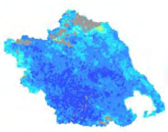
Χάρτης TVDI 2003_7_4
