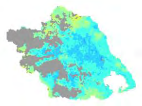
Χάρτης TVDI 2001_8_2
