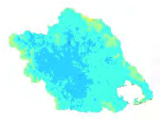
Χάρτης TVDI 2001_6_1
