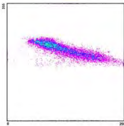
Διάγραμμα διασποράς 2005_6_2
