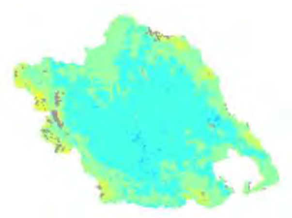
Χάρτης TVDI 2001_9_2
