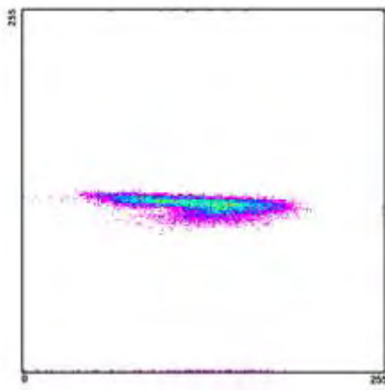
Διάγραμμα διασποράς 2002_11_3
