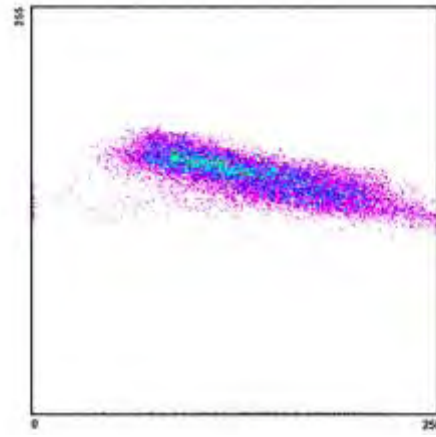
Διάγραμμα διασποράς 2005_5_3
