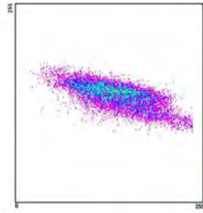
Διάγραμμα διασποράς 2003_9_1
