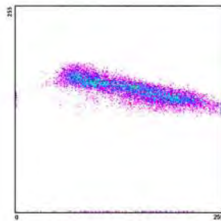
Διάγραμμα διασποράς 2004_6_1
