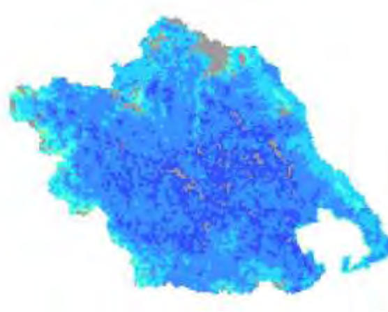
Χάρτης TVDI 2002_8_3
