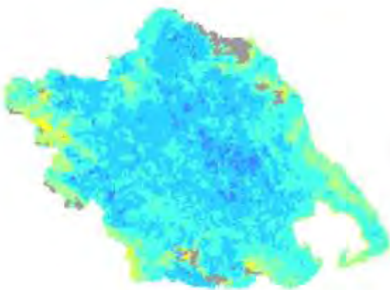
Χάρτης TVDI 2002_5_1
