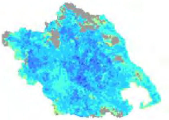
Χάρτης TVDI 2002_5_3
