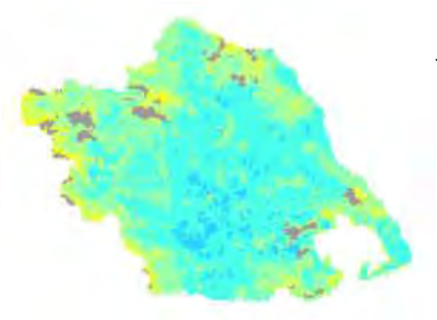
Χάρτης TVDI 2002_10_1
