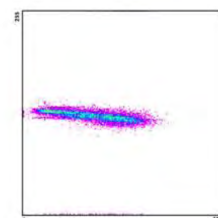
Διάγραμμα διασποράς 2004_11_1
