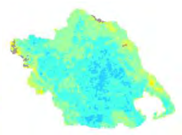
Χάρτης TVDI 2002_3_3
