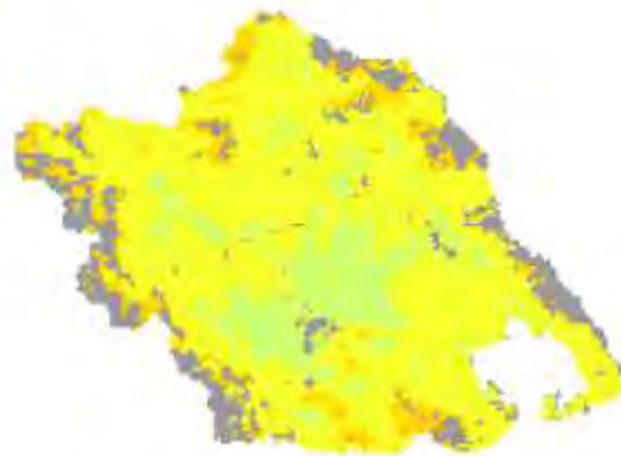
Χάρτης TVDI 2001_2_1
