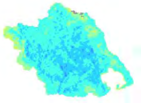
Χάρτης TVDI 2004_5_2
