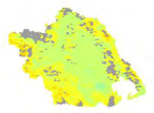
Χάρτης TVDI 2002_11_4
