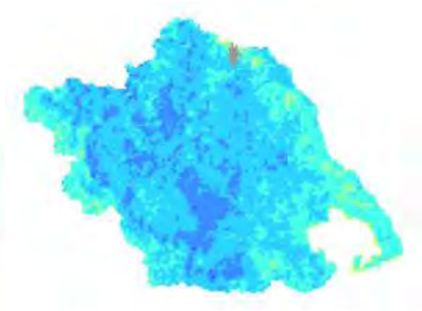
Χάρτης TVDI 2005_5_3
