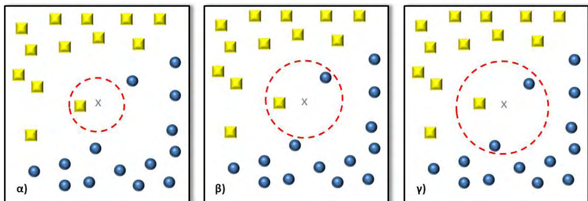
Εικόνα 3.1.2 Παράδειγμα επίλυσης προβλήματος με την χρήση του ταξινομητή k NN για α) k=1 , β) k=2 και γ) k=3 πλησιέστερους γείτονες.
