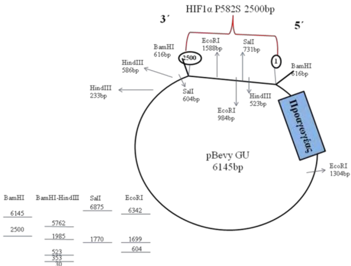
Διάγραμμα 2. Χάρτης πέψης του ανασυνδιασμένου πλασμιδίου pBenvy GU/HIF-1α από τα ενζύμα περιορισμού BamHI, HindIII, SalI και EcoRI. Το ένθεμα HIF-1α έχει κοινοποιηθεί με το σωστό προσανατολισμό.
