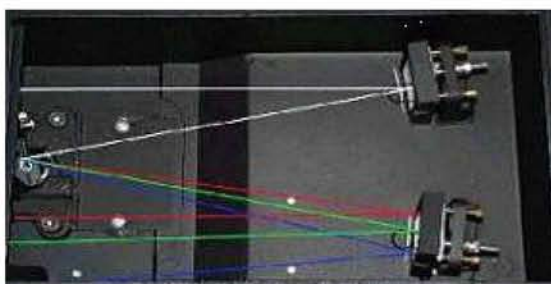
ΕΙΚΟΝΑ 9 Διάταξη FTIR με διαβαθμισμένο πλέγμα (grating).
