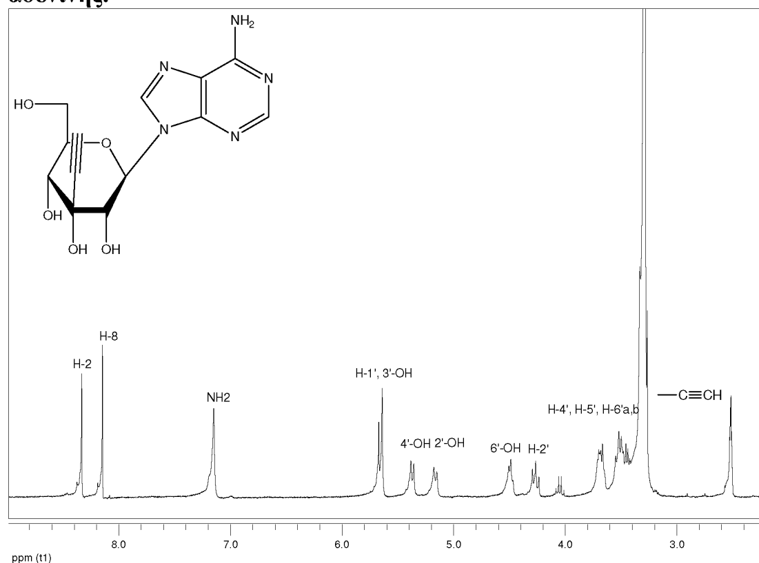
ΕΙΚΟΝΑ 16: Ταυτοποίηση της 9-(3'-C-αιθύνυλο-β-D-αλλοπυρανόζυλο) αδενίνης
