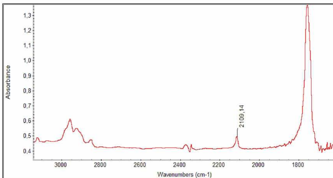
ΕΙΚΟΝΑ 15: Φάσμα υπερίθρου της 1-(3'-C-αιθυνυλο-β-D- αλλοπυρανοζυλο) κυτοσίνης
