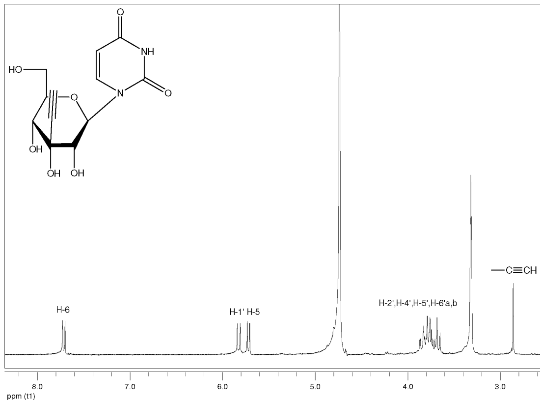
ΕΙΚΟΝΑ 12:Ταυτοποίηση της 1-(3'-C-αιθύνυλο-β-D-αλλοπυρανόζυλο) ουρακίλης
