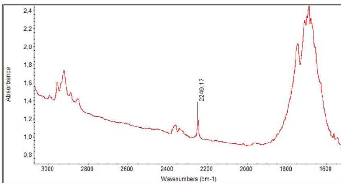
ΕΙΚΟΝΑ 19: Φάσμα υπερίθρου της 1-(3'-C-αιθύνυλο-β-D-αλλοπυρανόζυλο) 5-φθοροουρακίλης
