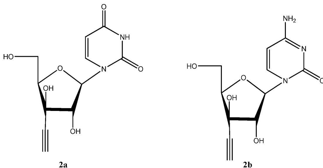
Σχήμα 4. 3'έπιμερή των ECyd και EUrd
