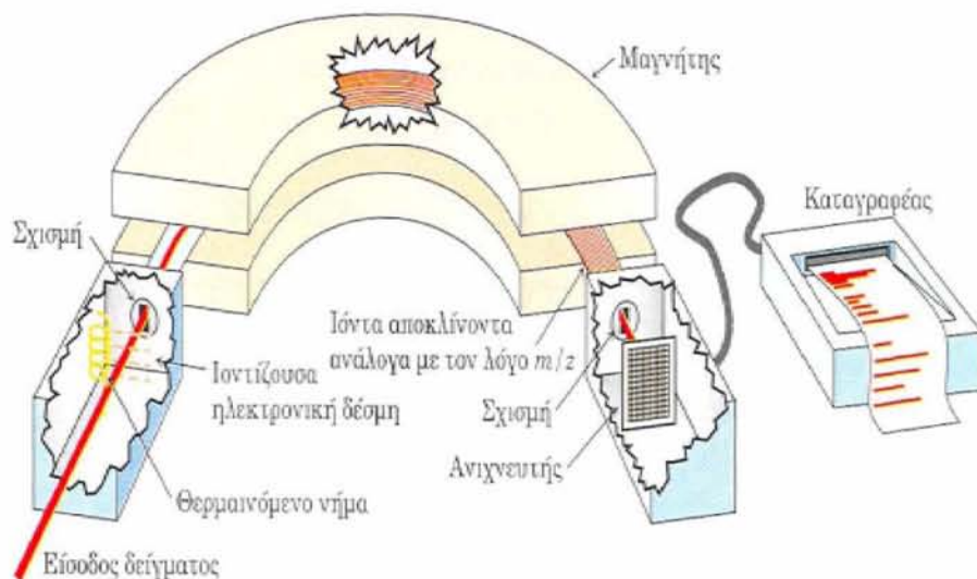
ΕΙΚΟΝΑ 1 Φασματόμετρο Μάζας
