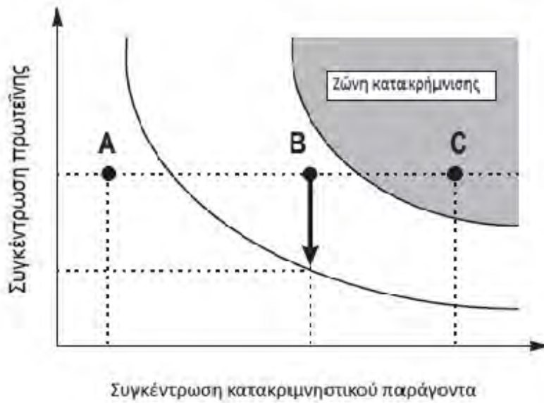
Εικόνα 6 Διάγραμμα φάσης για τη μέθοδο micro – batch
