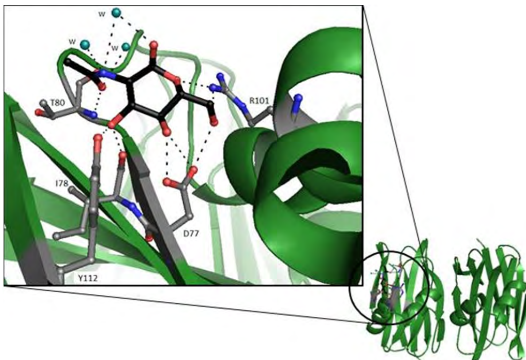
Εικόνα 36 Η θέση σύνδεσης του 2-Acetylamino-2-Deoxy-Alpha-D-Mannopyranose στη δεύτερη υπομονάδα της SSR1, και οι δεσμοί υδρογόνου που σχηματίζει με μόρια νερού(w) και αμινοξικά κατάλοιπα στη θέση αυτή.
