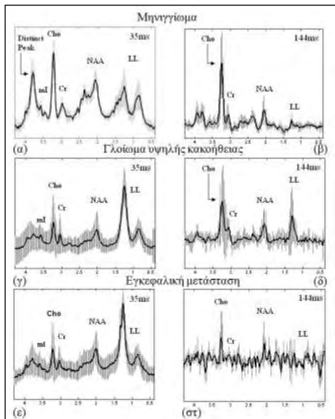
Εικόνα 5.2.2: Τα μέσα φάσματα και οι αντίστοιχες τυπικές αποκλίσεις των μηνιγγιωμάτων (α, β), γλοιωμάτων υψηλής κακοήθειας (γ, δ) και των εγκεφαλικών μεταστάσεων (ε, στ), όπως υπολογίστηκαν για χαμηλό (α, γ, ε) και υψηλό (β, δ, στ) χρόνο ηχούς.
