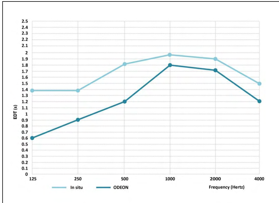
Πίνακας 11: Early Decay Time (EDT) – Κυλικείο (In situ/ODEON)
