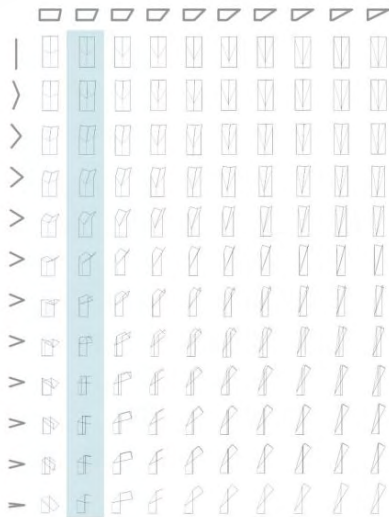
Πίνακας 7.2: Διαγραμματικός πίνακας με τις σταδιακές αλλαγές του βαθμού κλίσης ( \alpha ) μίας μονής αντίστροφης πτύκωσης ('miura'- 'yoshimura') και τα αντίστοιχα στάδια αναδίπλωσής της (δ). (Rigid Origami Simulator)
