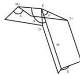
Πίνακας 7.2: Διαγραμματικός πίνακας με τις σταδιακές αλλαγές του βαθμού κλίσης ( \alpha ) μίας μονής αντίστροφης πτύκωσης ('miura'- 'yoshimura') και τα αντίστοιχα στάδια αναδίπλωσής της (δ). (Rigid Origami Simulator)
