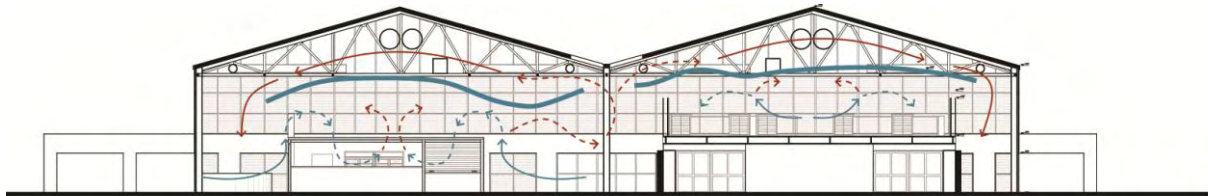
ΤΟΜΗ ΧΩΡΟΥ ΕΠΕΜΒΑΣΗΣ-ΔΙΑΓΡΑΜΜΑ ΨΥΞΗΣ/ΘΕΡΜΑΝΣΗΣ (ΘΕΡΙΝΗ ΠΕΡΙΟΔΟΣ)
