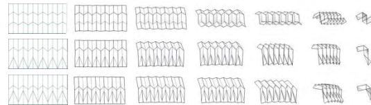
Εικόνα 11.1: Στάδια μορφολογικής εξέλιξης του αρχικού 'origami pattern' μετά την εφαρμογή των γεωμετρικών μετατροπών που προαναφέρθηκαν (αλλαγή γωνίας αναδίπλωσης των πτυχώσεων, αλλαγή αποστάσεων μεταξύ των οριζόντιων 'γραμμών' πτυχώσεων).
