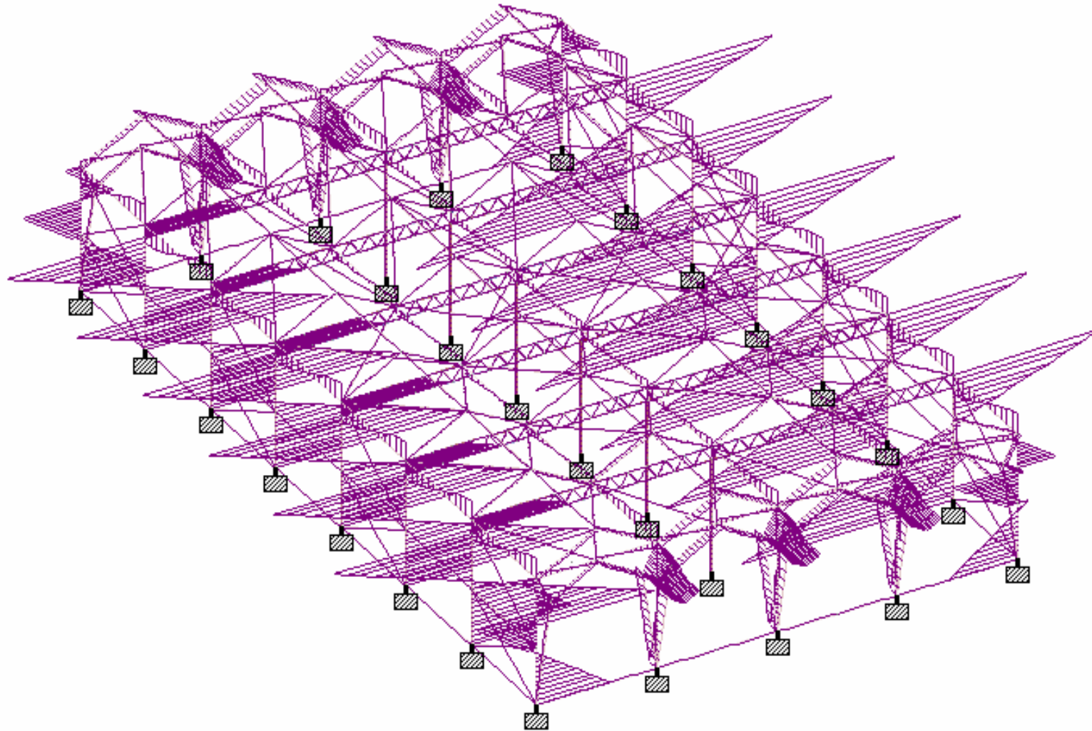
Ενδεικτικό διάγραμμα τενουσών δυνάμεων [Qz]
