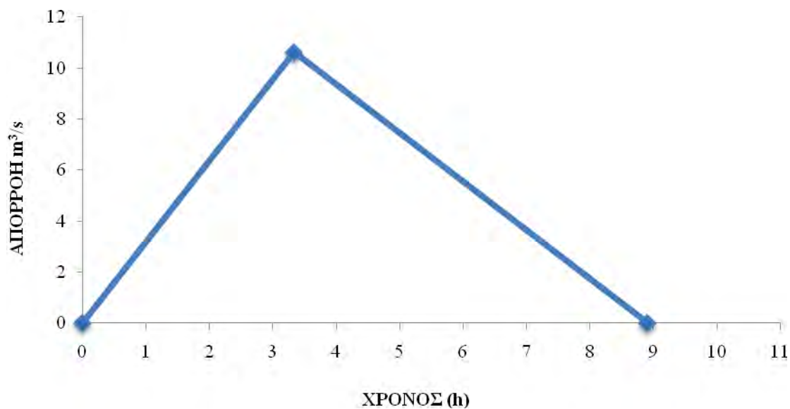
Σχήμα 14: Τριγωνικό υδρογράφημα της μεθόδου S.C.S.
