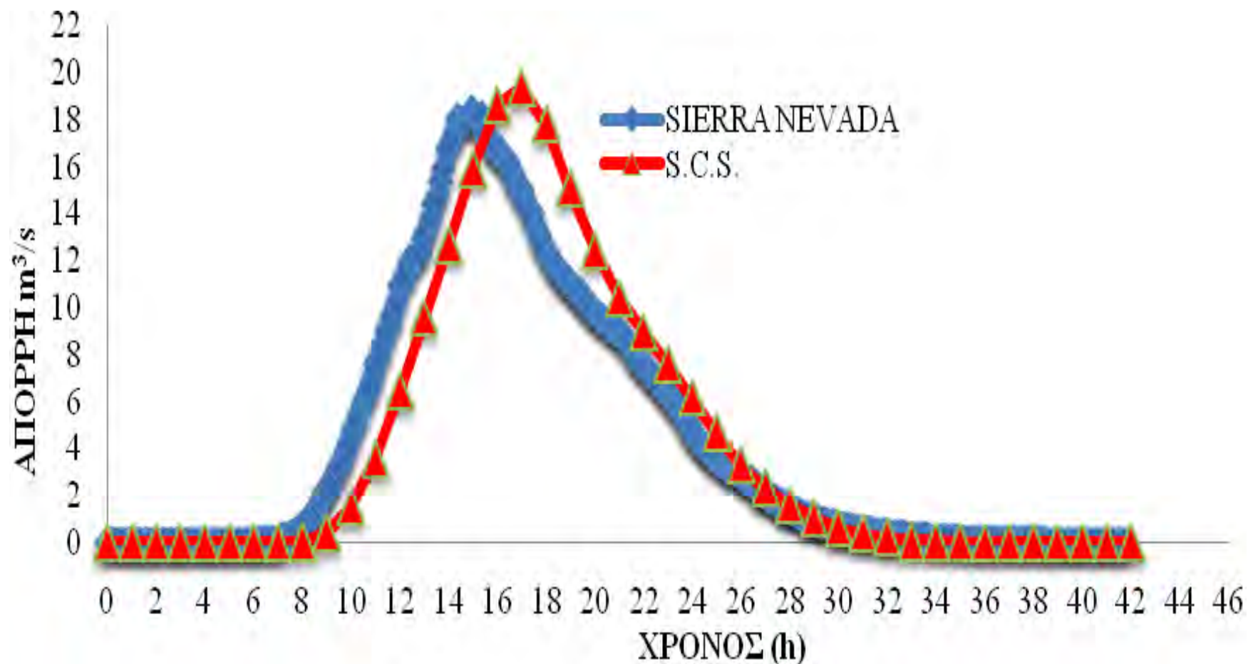
Σχήμα 35: Υδρογραφήματα πλημμύρας.
