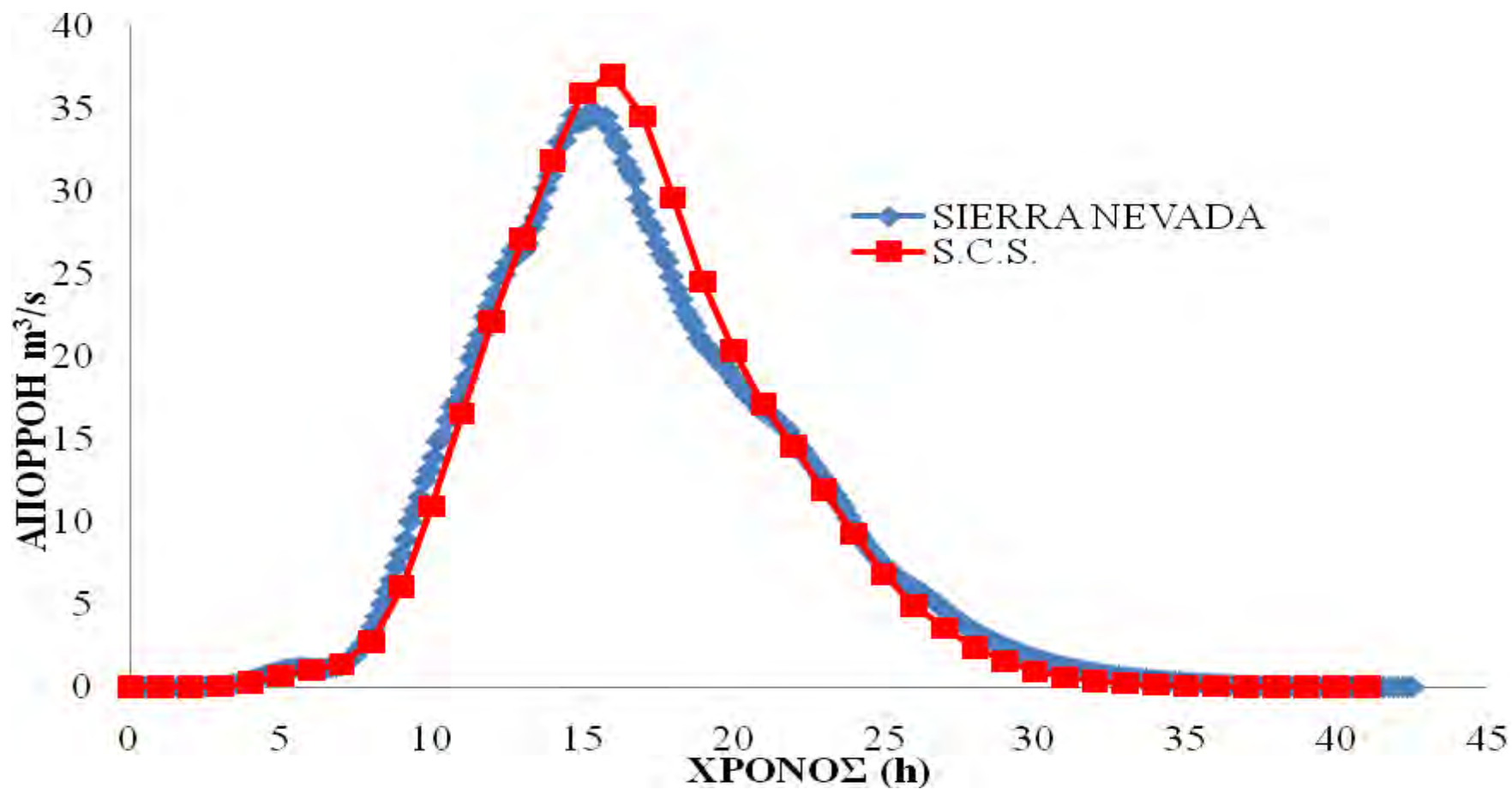
Σχήμα 24: Υδρογραφήματα πλημμύρας.
