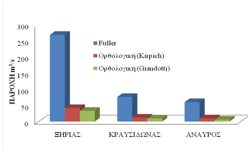
Σχήμα 38: Σύγκριση πλημμυρικών παροχών για περίοδο επαναφοράς T = 20
