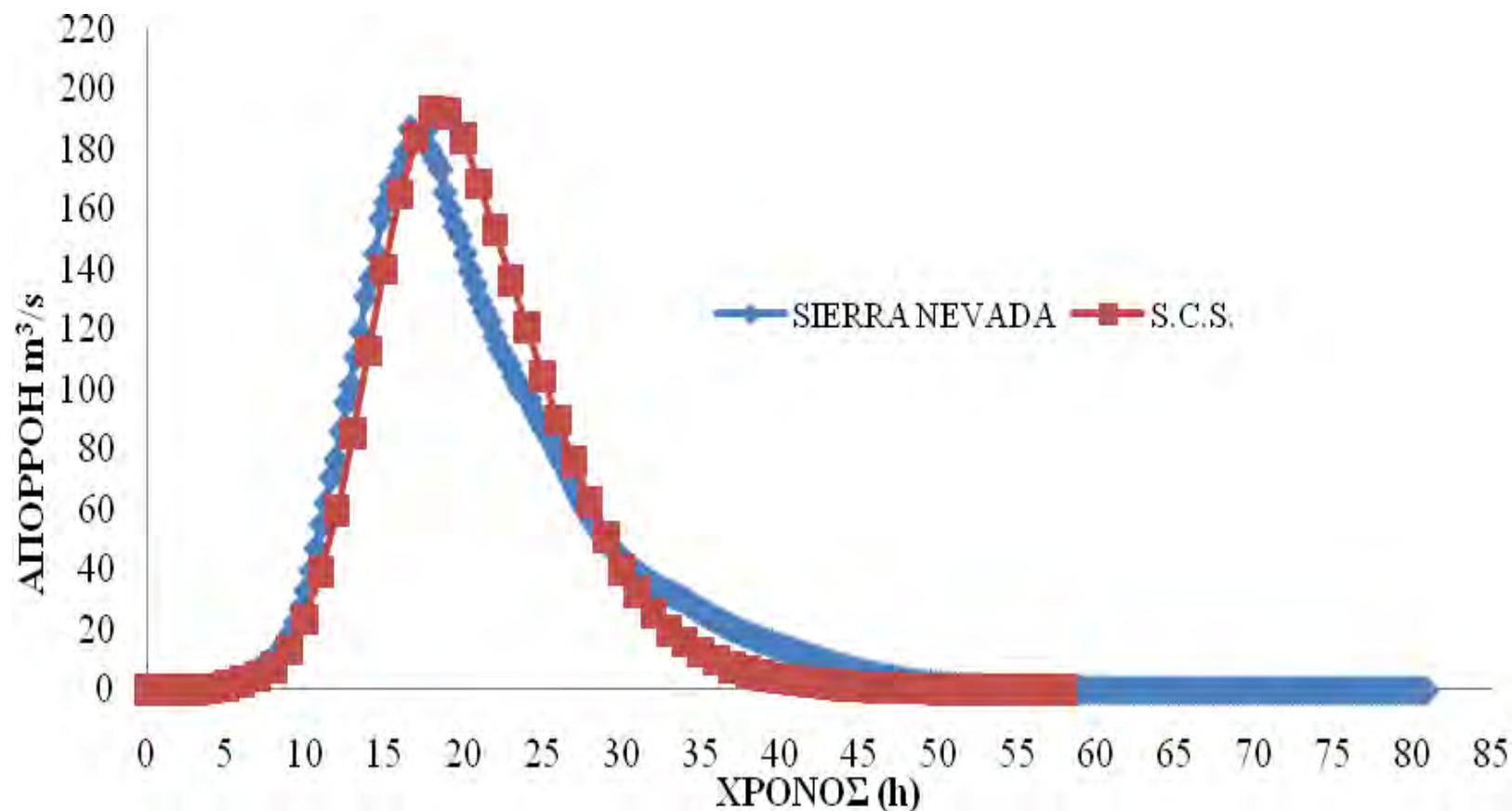
Σχήμα 13: Υδρογραφήματα.
