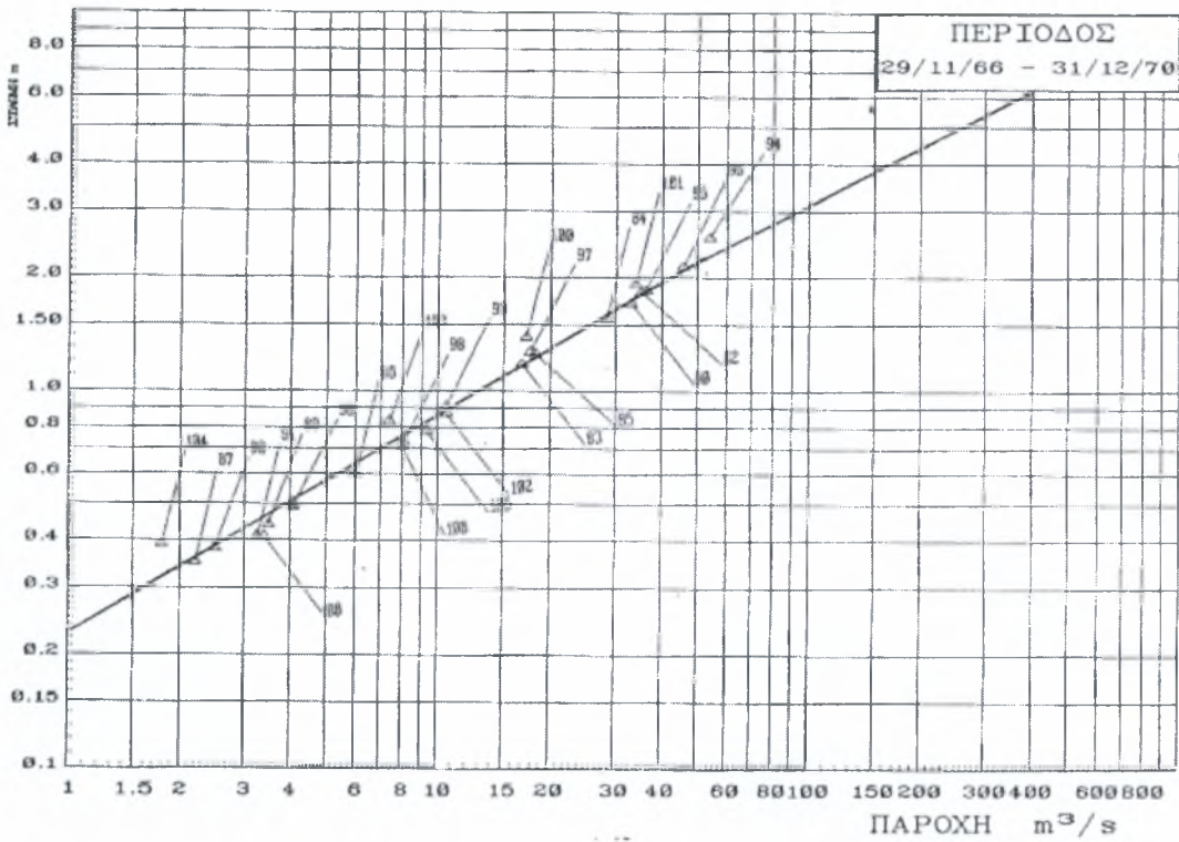
ΚΑΜΠΥΛΕΣ ΣΤΑΘΜΗΣ ΠΑΡΟΧΗΣ ΓΕΦ. ΚΟΜΠΟΤΑΔΩΝ ΣΠΕΡΧΕΙΟΥ
