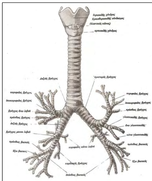
Εικόνα 1. Εντοπισμός του λάρυγγα, της τραχείας, και του βρογχικού δέντρου του αναπνευστικού συστήματος (Ανατύπωση από: Αλεξάνδρου Π. Σάββα, Επιτομή, ανατομική του ανθρώπου και Άτλας, Δ' έκδοση, κεφάλαιο Αναπνευστικού συστήματος, Εκδοτικός οίκος αφών Κυριακίδη, Θεσσαλονίκη 1989).
