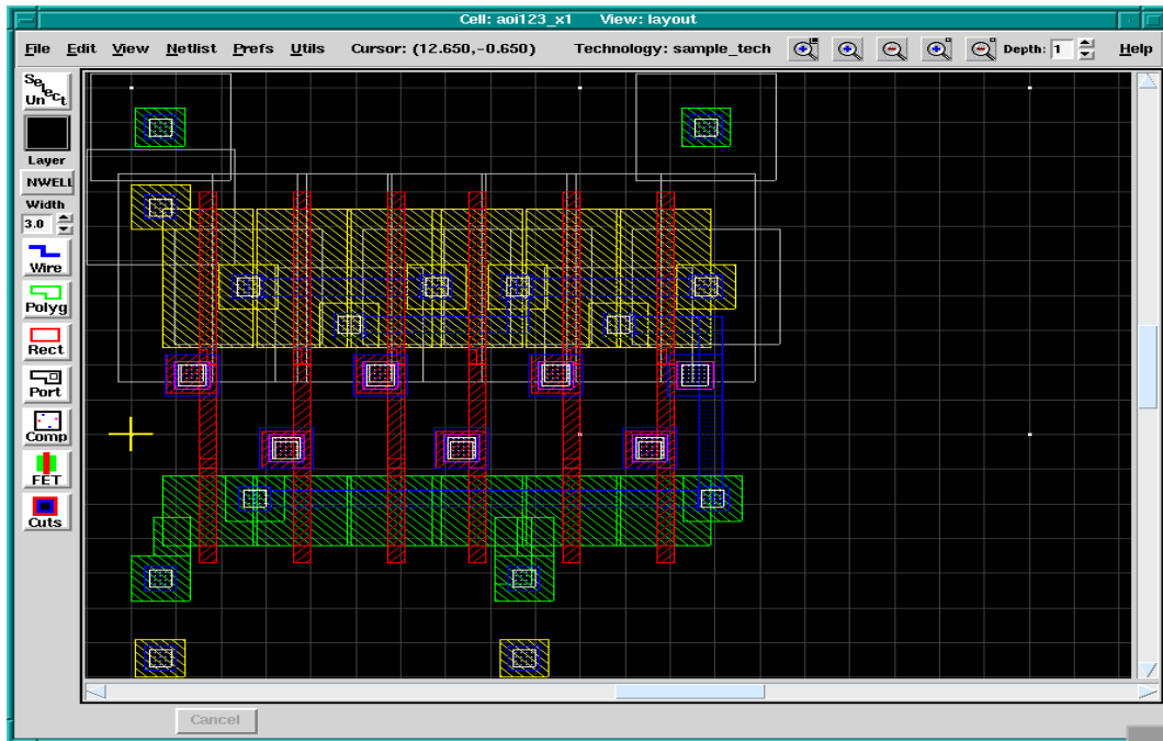
Εικόνα 2.3: Αναπαράσταση ενός Standard cell Layout
