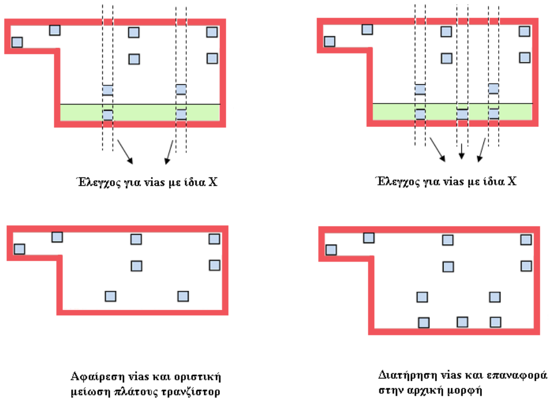
Εικόνα 5.12: Έλεγχος για αφαίρεση vias και για οριστική μείωση του πλάτους των τρανζίστορ.
