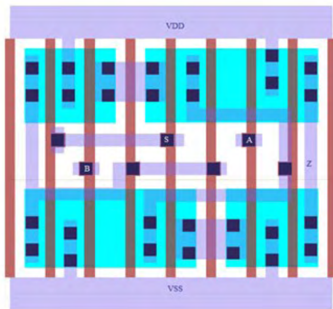
Εικόνα 2.2: Παράδειγμα Standard Cell Layout
