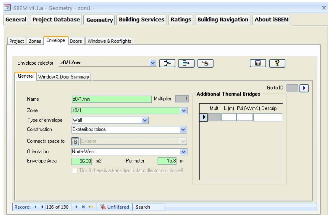
Εικόνα 30: Η υπο-ετικέτα Γενικά της ετικέτας Κέλυφος
