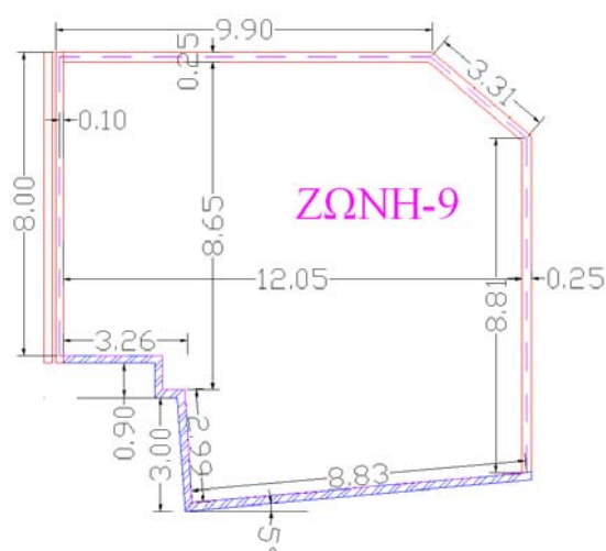
Εικόνα 75. Κάτοψη ζώνης 9 στο ισόγειο.
