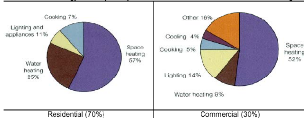
Εικόνα 3. Η κατανάλωση ενέργειας στα κτίρια [8]
