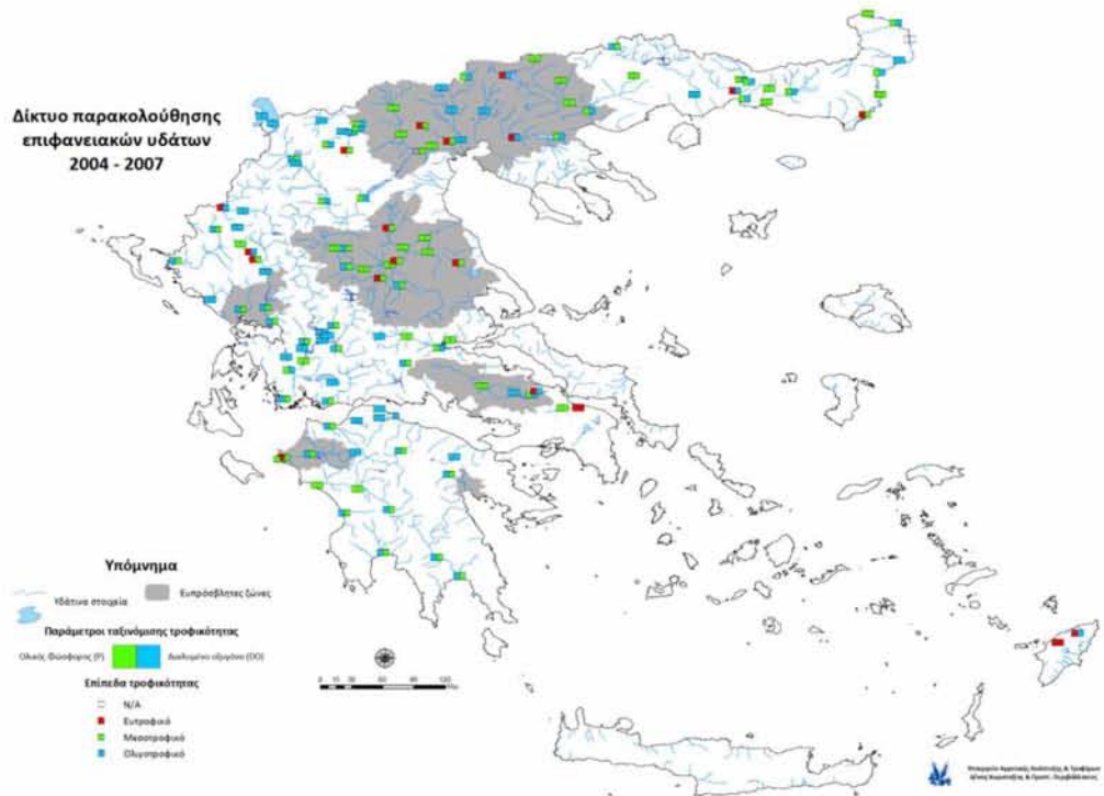
Χάρτης 13: Χαρακτηρισμός επιφανειακών υδάτων ως προς την τροφική τους κατάσταση με βάση τις συγκεντρώσεις ολικού φωσφόρου και διαλυμένου οξυγόνου (Πηγή: www.minargic.gr )
