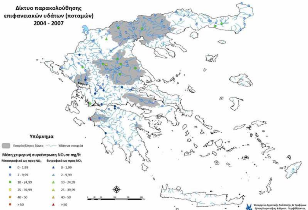
Χάρτης 12: Μέση χειμερινή συγκέντρωση νιτρικών των επιφανειακών υδάτων χαρακτηρισμένα ως μεσοτροφικά και ευτροφικά ως προς NO 3 (Πηγή: www.minagric.gr )
