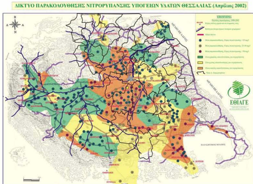
Χάρτης 6: Δίκτυο παρακολούθησης νιτρορύπανσης υπογείων υδάτων Θεσσαλίας
