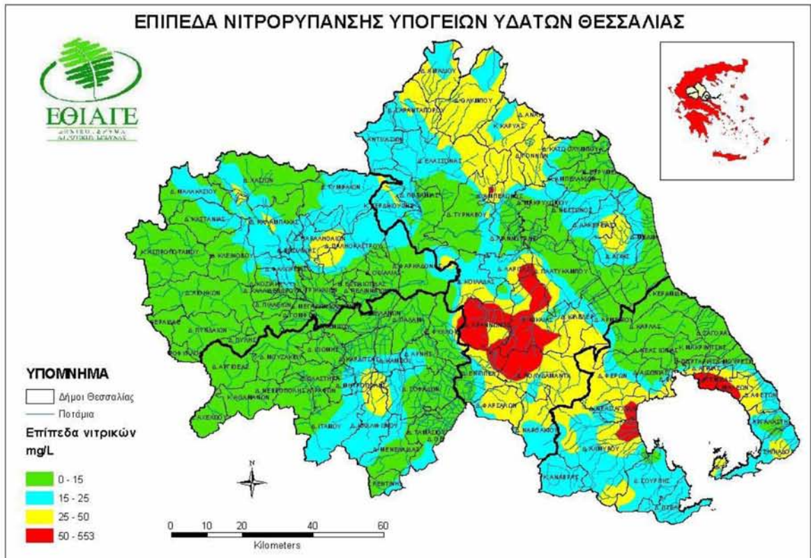
Χάρτης 5: Επίπεδα νιτρορύπανσης υπογείων υδάτων Θεσσαλίας
