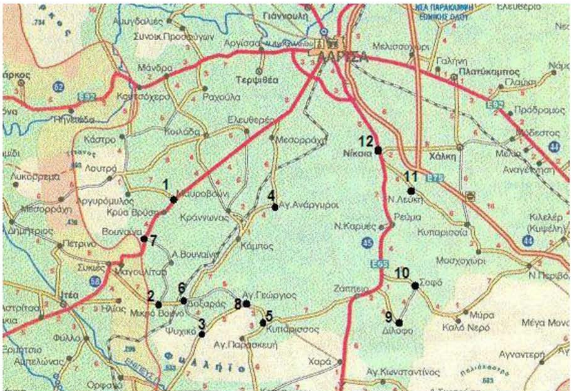
Χάρτης 3: Σταθμοί δειγματοληψίας
