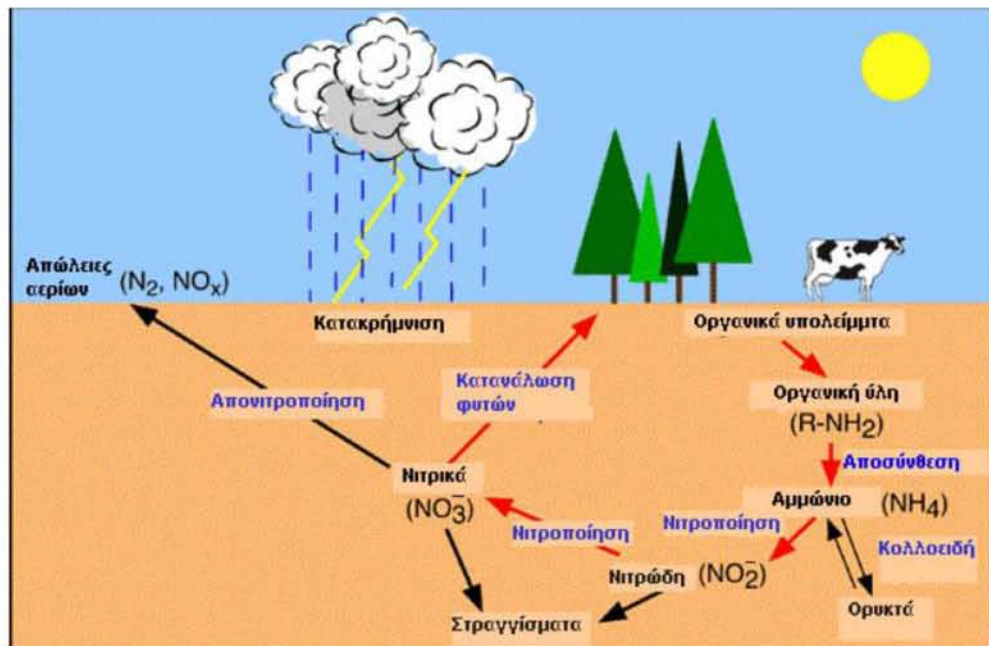
Σχήμα 4: Ο κύκλος του αζώτου (Πηγή: Τσαουσιδου, 2008)
