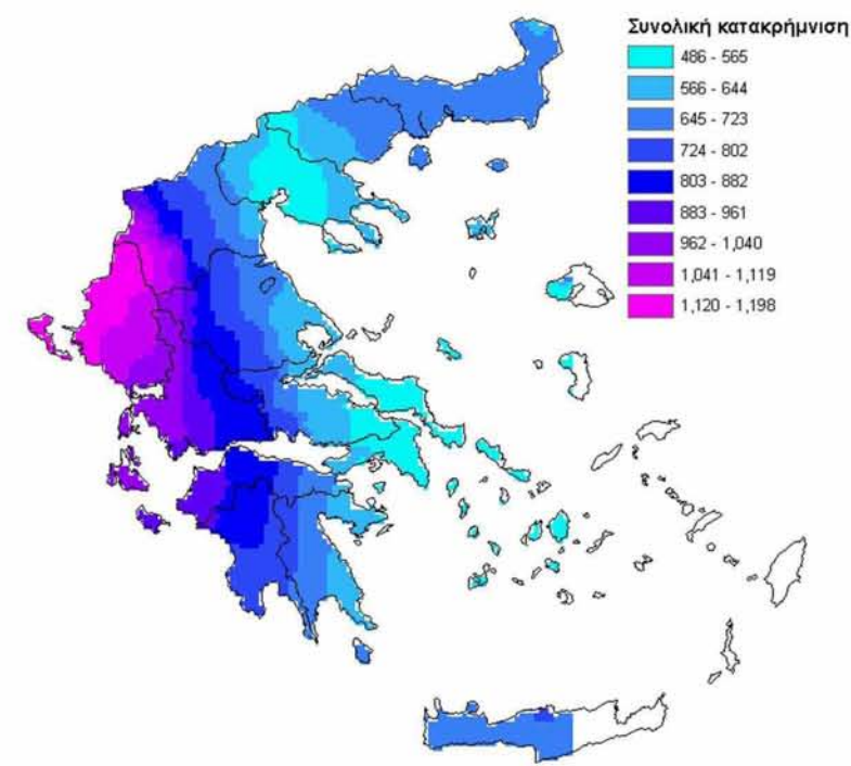
Χάρτης 1: Συνολική κατακρήμιση στην Ελλάδα (Πηγή: http://ndbhmi.chi.civil.ntua.gr )
