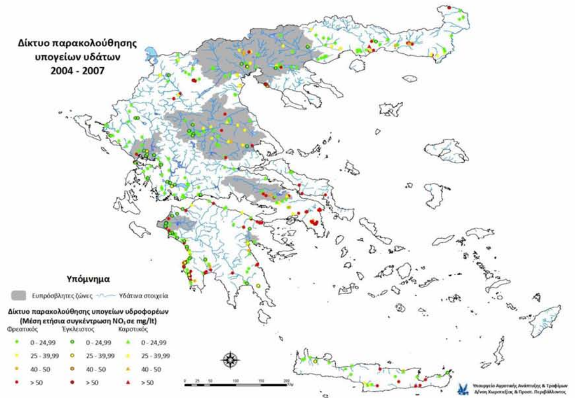
Χάρτης 14: Μέση ετήσια συγκέντρωση νιτρικών στο δίκτυο παρακολούθησης των υπογείων υδάτων για την περίοδο 2004 – 2007 κατά κατηγορία υπόγειου υδροφορέα. (Πηγή: www.minargic.gr )
