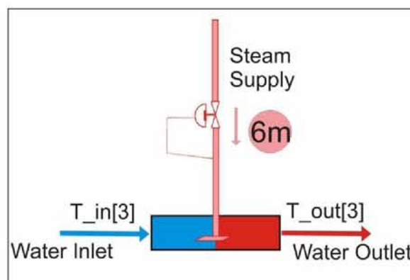
Σχήμα 22: Διάγραμμα ροών συσκευών ανάμειξης
