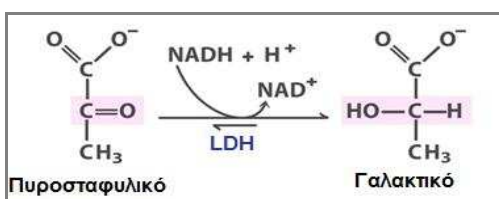
Εικόνα 6: Μετατροπή του πυροσταφυλικού σε γαλακτικό οξύ από τη γαλακτική δεϋδρογονάση (LDH).
