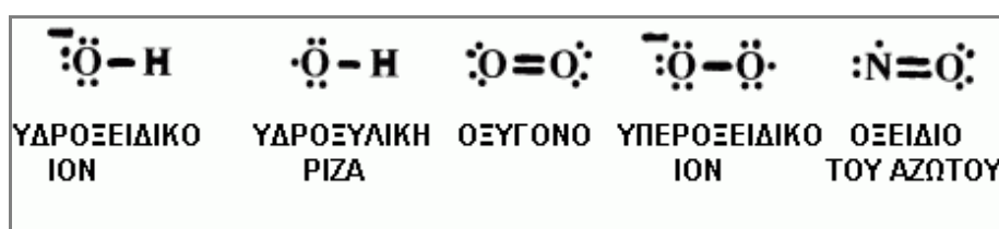
Εικόνα 52: Ηλεκτρονιακή κατάσταση της εξωτερικής στοιβάδας των διαφόρων δραστικών μορφών αζώτου και οξυγόνου.
