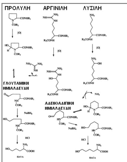
Εικόνα 70: Σχήμα αντίδρασης της δημιουργίας των γλουταμινικών και αμινοαδιπικών ημιαλδευδών. Τα κύρια προϊόντα της καταλύμενης οξειδωσης μέσω μετάλων της πολυαργινίνης και της πολυπρολίνης (γλουταμικής ημιαλδεύδης) και της πολυλυσίνης (αμινοαδιπικής ημιαλδεύδης).
