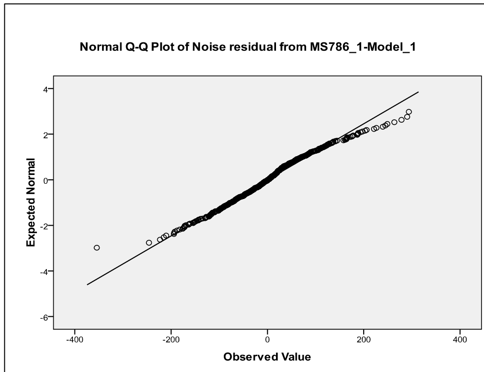
Σχήμα 6.11: Q-Q plot των καταλοίπων του πολυμεταβλητού μοντέλου
