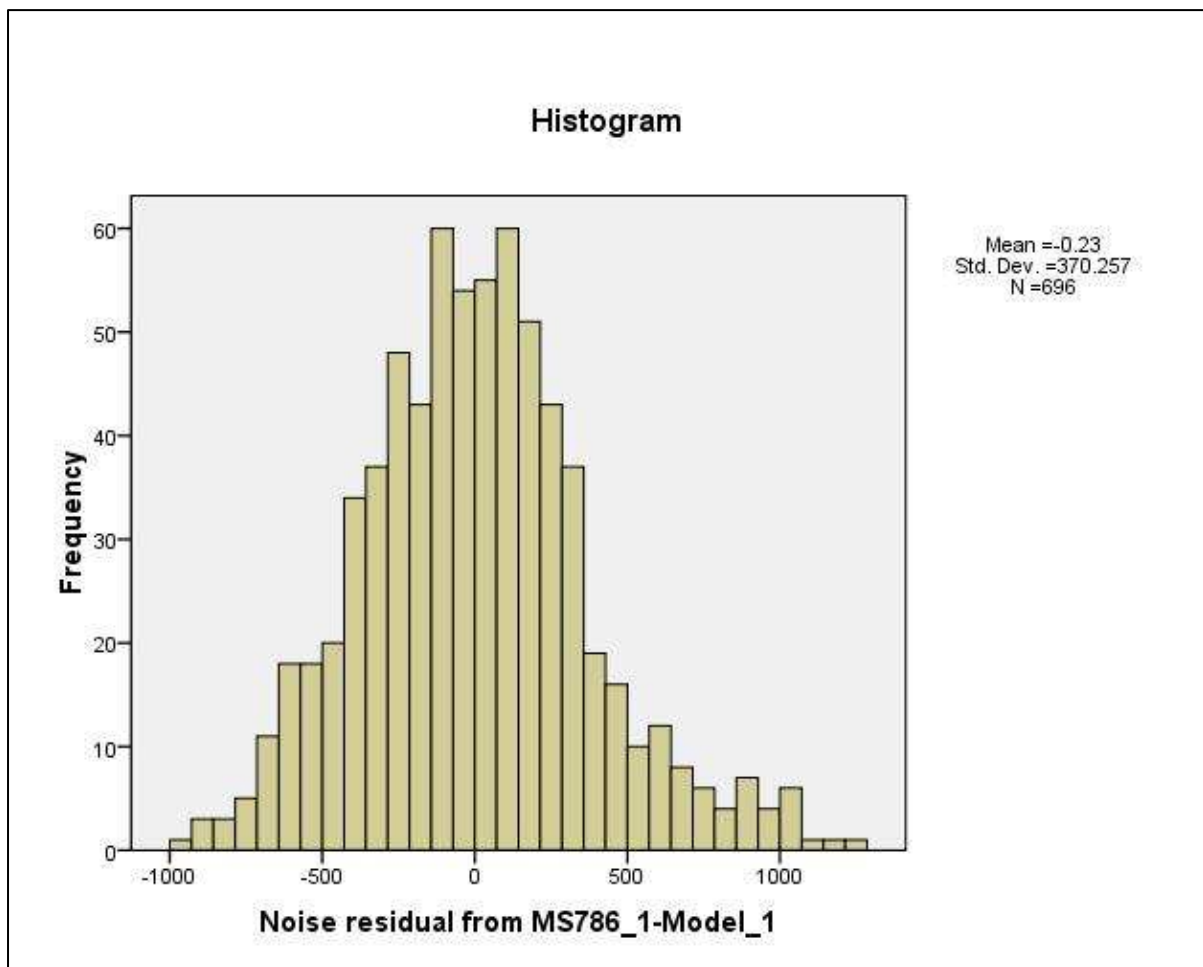
Σχήμα 6.4: Ιστογράμμα κατανομής καταλοίπων του μονομεταβλητού μοντέλου
