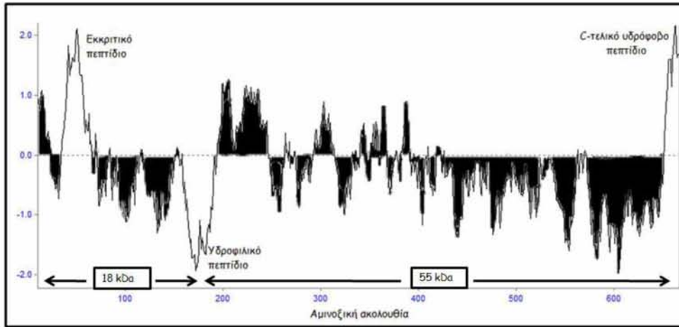
Εικόνα 3-18: Προφίλ υδροφοβικότητας της αμινοξικής ακολουθίας της ακετυλοχολινεστεράσης του δάκου όπως προκύπτει από το πρόγραμμα Ompa 2.0 (Oxford Molecular Ltd). Οι θετικές τιμές του άξονα Y υποδεικνύουν την υδροφοβικότητα της πρωτεΐνης, ενώ αντίθετα οι αρνητικές τιμές την υδροφιλικότητα. Το εκκριτικό πεπτιδίο, το υδροφιλικό πεπτιδίο υπεύθυνο για το διαχωρισμό των δύο υπομονάδων (18 kDa, 55 kDa) και το καρβοξυτελικό υδρόφοβο πεπτιδίο που σηματοδοτεί την προσθήκη GPI άγκυρας υποδεικνύονται με τις λευκές περιοχές. Το γράφημα έγινε με τη μέθοδο των Kyte & Doolittle (1982).
