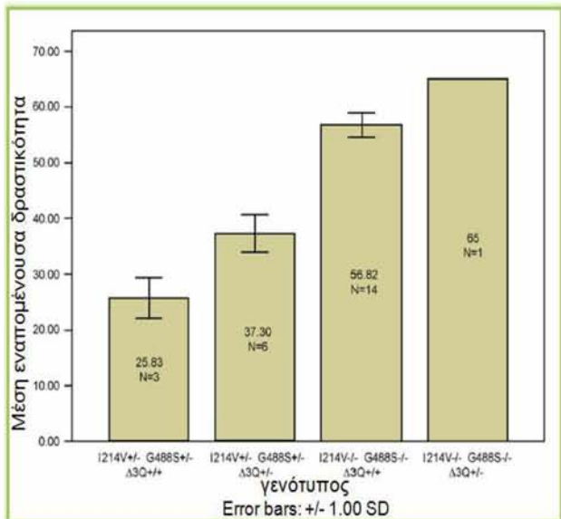
Εικόνα 3-38: Η εναπομένουσα δραστικότητα της ακετυλοχολινεστεράσης (ύστερα από αναστολή με εντομοκτόνο) των διαφορετικών γενοτύπων του γονιδίου της ακετυλοχολινεστεράσης του δάκου. Η γραφική παράσταση προήλθε από το πρόγραμμα στατιστικής ανάλυσης SPSS 13.0 for Windows (Leadtools). Μέσα στις στήλες εμφανίζεται η τιμή της μέσης εναπομένουσας δραστικότητας του ενζύμου και ο αριθμός των ατόμων (N) που ελέγχθηκαν. Η τυπική απόκλιση (error bars) παρουσιάζεται στην κορυφή των στηλών.
