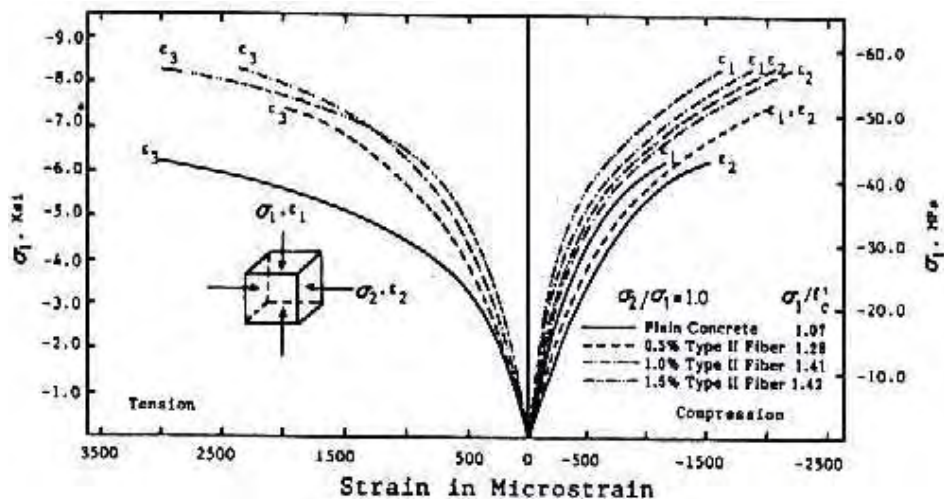
Σχήμα 23. ΚΑΜΠΥΛΕΣ ΤΑΣΕΩΝ-ΠΑΡΑΜΟΡΦΩΣΕΩΝ ΓΙΑ ΛΟΙΠΟ ΚΑΙ ΙΝΟΠΛΙΣΜΕΝΟ ΣΚΥΡΟΔΕΜΑ (ΙΝΕΣ ΤΥΠΟΥ II) ΥΠΟ ΔΙΑΞΟΝΙΚΗ ΘΛΙΨΗ.
