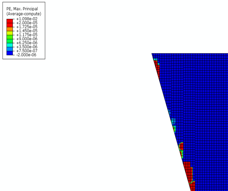
Σχήμα 60. ΚΑΤΑΝΟΜΗ ΤΗΣ ΠΛΑΣΤΙΚΗΣ ΚΥΡΙΑΣ ΜΕΓΙΣΤΗΣ ΠΑΡΑΜΟΡΦΩΣΗΣ ΣΤΗΝ ΠΛΑΚΑ ΤΟΥ ΦΡΑΓΜΑΤΟΣ, ΜΕΤΑ ΤΗΝ ΠΛΗΡΩΣΗ ΤΗΣ ΛΕΚΑΝΗΣ. ΣΚΥΡΟΔΕΜΑ C25, ΙΝΟΠΛΙΣΜΕΝΟ, ΚΑΝΟΝΙΚΟΣ ΟΠΛΙΣΜΟΣ Φ36/20.
