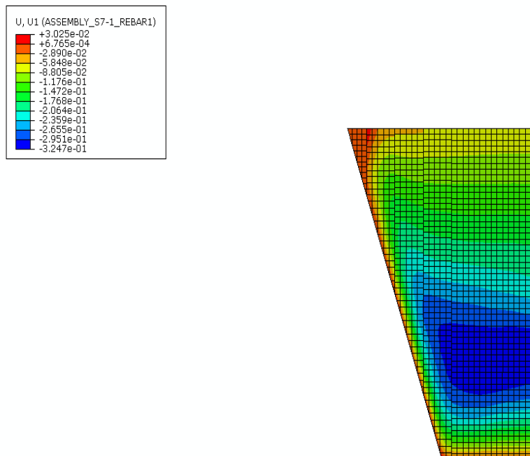
Σχήμα 66. ΚΑΤΑΝΟΜΗ ΤΗΣ ΒΥΘΙΣΗΣ ΣΤΗΝ ΠΛΑΚΑ ΤΟΥ ΦΡΑΓΜΑΤΟΣ, ΜΕΤΑ ΤΗΝ ΠΛΗΡΩΣΗ ΤΗΣ ΛΕΚΑΝΗΣ. ΣΚΥΡΟΔΕΜΑ C37, ΙΝΟΠΛΙΣΜΕΝΟ, ΚΑΝΟΝΙΚΟΣ ΟΠΛΙΣΜΟΣ \Phi 36/20 .
